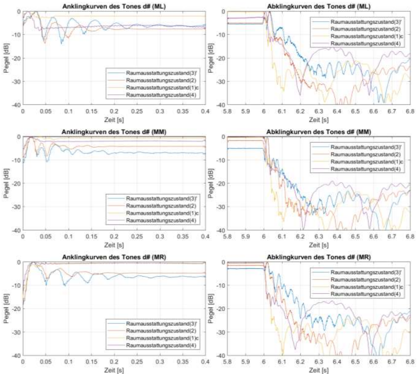
Abb. B1.16: An- und Abklingkurven der Marimbatonmessungen bei Anregung von Quellposition (Q2) mit der Grundfrequenz des Tones d# ( \triangleq 157 Hz) für alle vier Raumausstattungs Zustände (3)', (2), (1)c und (4) sowie die Mikrofonpositionen (ML), (MM) und (MR)
