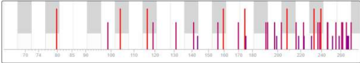
Abb. 3.1: Moden der Übekabine mit hinterlegter Klaviatur ( a' = 443 Hz) im Bereich von C bis 280 Hz ( \cong c\sharp' ) [ https://trikustik.at/raummoden-rechner/ (22.08.2018)]
