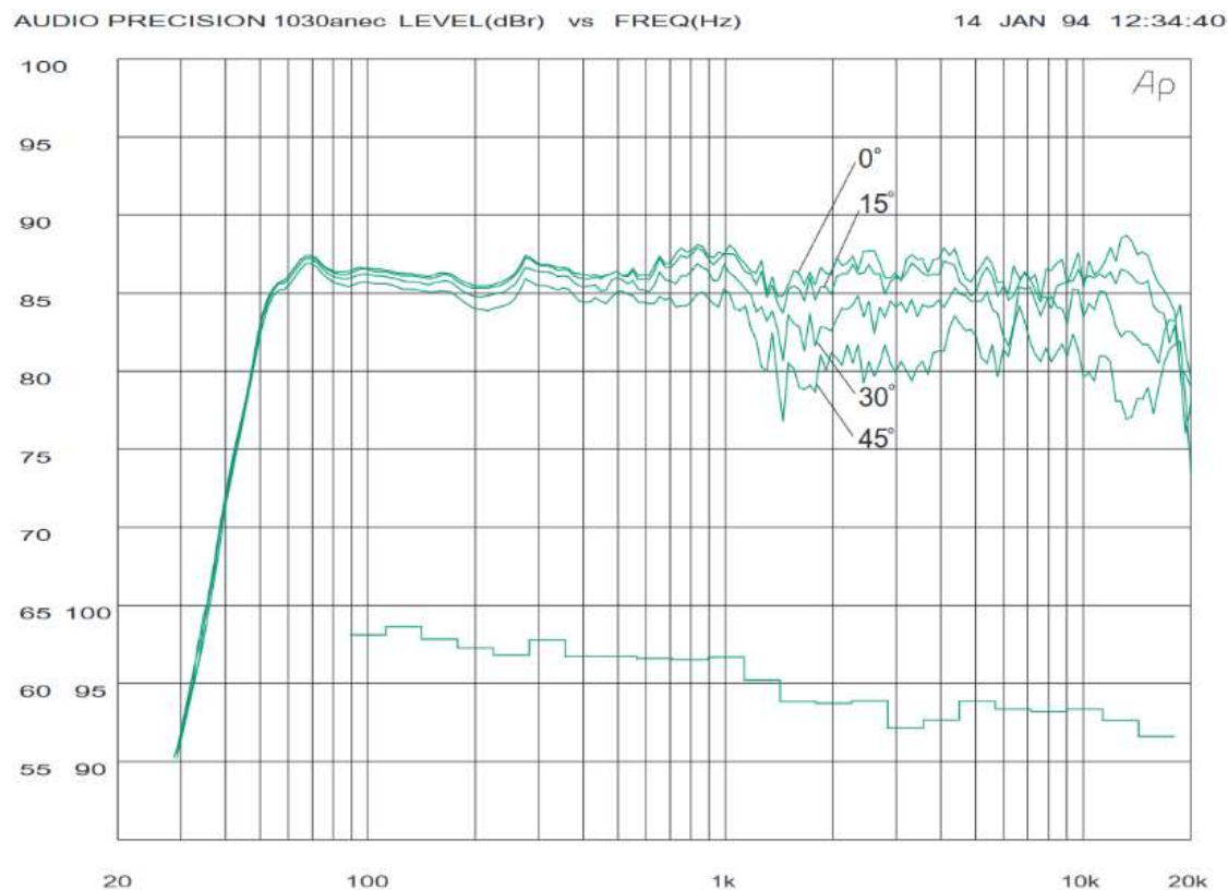
Abb. 4.1: Richtungsabhängiger SPL-Verlauf des vertikal platzierten Genelec 1030A Studiomonitors in 1 m Entfernung [oben] und terzbandgefilterter Schallleistungsverlauf [unten] aus Herstellerdatenblatt [ https://www.genelec.com/sites/default/files/media/Previous%20models/2-way%20loudspeakers/1030A/ds1030a.pdf ] (14.10.2018)]
