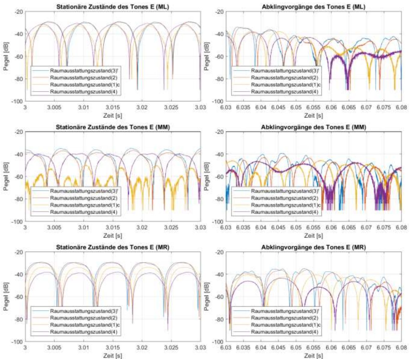
Abb. B2.5: Messsignalwellenformen der Marimbatonmessungen bei Anregung von Quellposition ( Q1 ) mit der Grundfrequenz des Tones E ( \cong 83 Hz) für alle vier Raumausstattungs Zustände ( 3' ), ( 2 ), ( 1c ) und ( 4 ) sowie die Mikrofonpositionen ( ML ), ( MM ) und ( MR )
