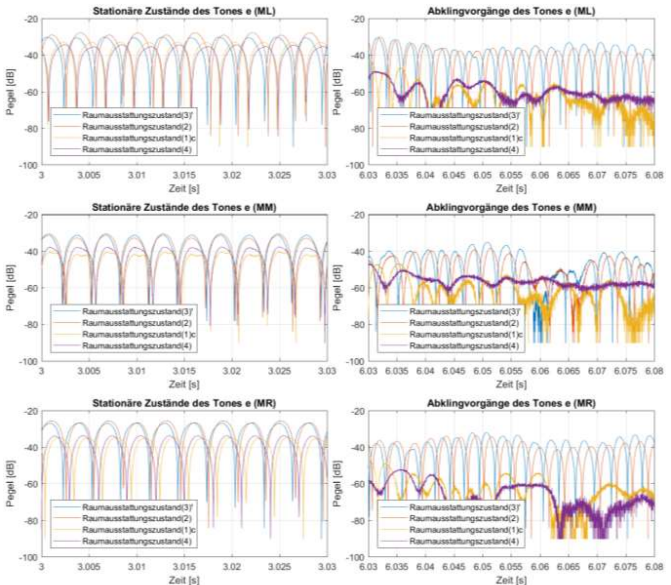
Abb. B2.17: Messsignalwellenformen der Marimbatonmessungen bei Anregung von Quellposition (Q2) mit der Grundfrequenz des Tones e ( \approx 166 Hz) für alle vier Raumausstattungs Zustände (3) f , (2), (1)c und (4) sowie die Mikrofonpositionen (ML), (MM) und (MR)
