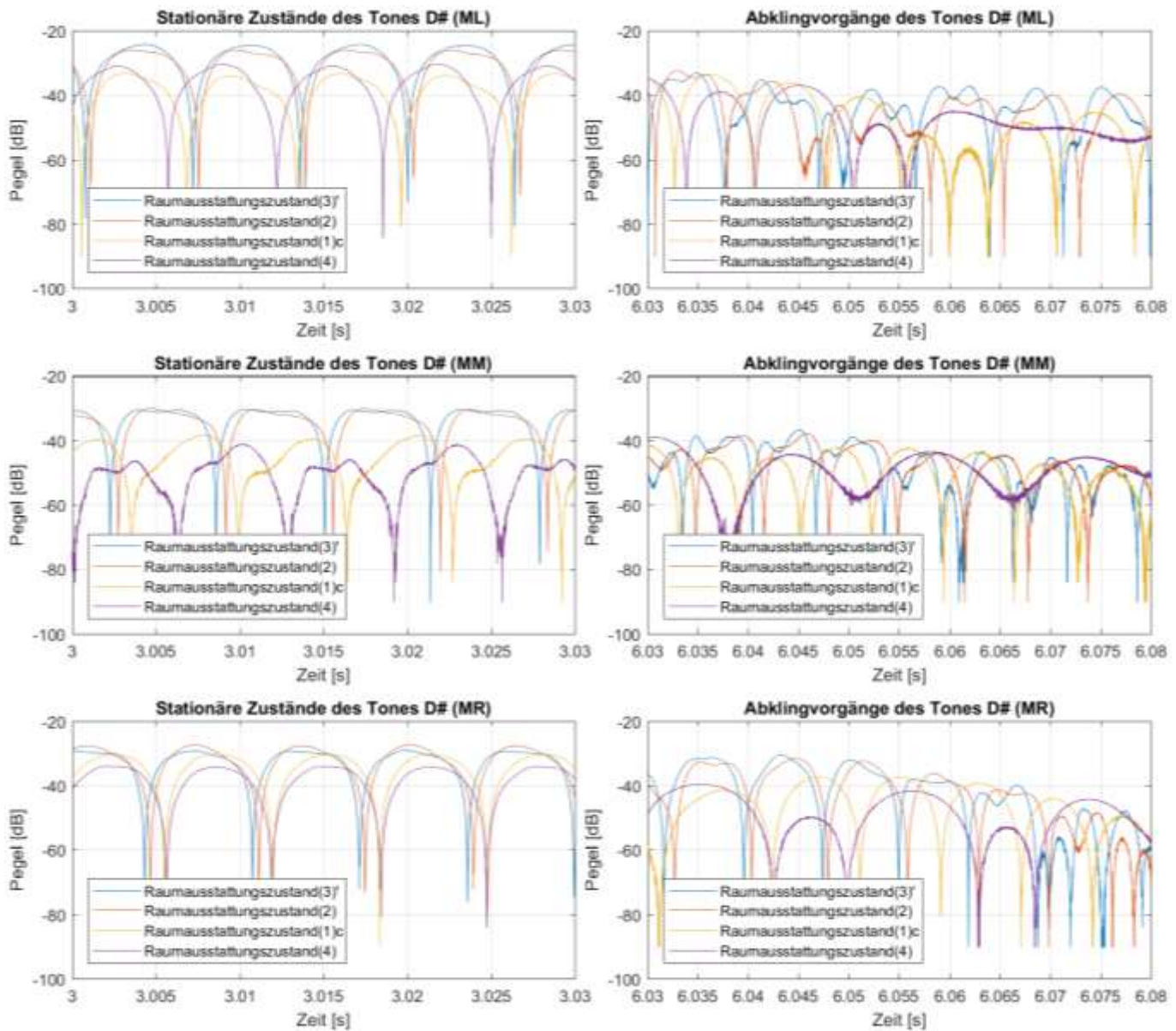
Abb. B2.4: Messsignalwellenformen der Marimbatonmessungen bei Anregung von Quellposition (Q1) mit der Grundfrequenz des Tones D# ( \cong 78 Hz) für alle vier Raumausstattungs Zustände (3) * , (2), (1)c und (4) sowie die Mikrofonpositionen (ML), (MM) und (MR)
