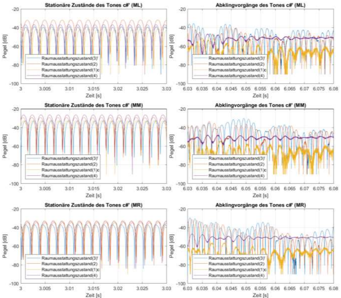
Abb. B2.26: Messsignalwellenformen der Marimbatonmessungen bei Anregung von Quellposition (Q3) mit der Grundfrequenz des Tones c# ( \approx 279 Hz) für alle vier Raumausstattungs Zustände (3) f , (2), (1)c und (4) sowie die Mikrofonpositionen (ML), (MM) und (MR)
