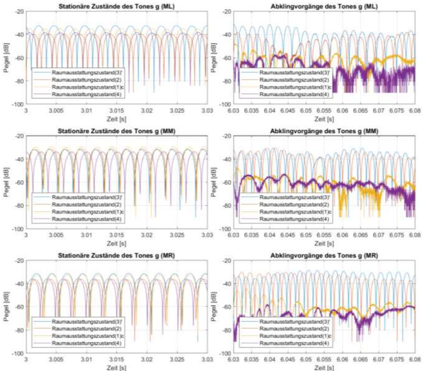
Abb. B2.20: Messsignalwellenformen der Marimbatonmessungen bei Anregung von Quellposition (Q3) mit der Grundfrequenz des Tones g ( \approx 197 Hz) für alle vier Raumausstattungszustände (3) * , (2), (1)c und (4) sowie die Mikrofonpositionen (ML), (MM) und (MR)
