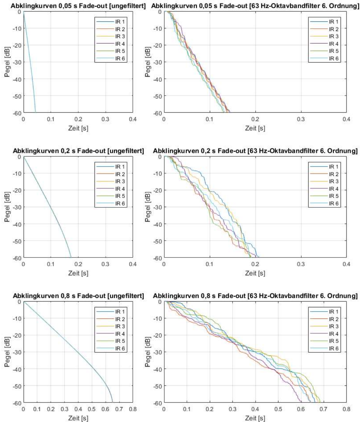
Abb. 5.16: Abklingkurven der ungefilterten sowie der mit dem 63 Hz-Oktavbandfilter 6. Ordnung gefilterten unterschiedlichen Pseudoransch-Impulsantworten mit 0,05 s, 0,2 s und 0,8 s Fade-out-Dauer
