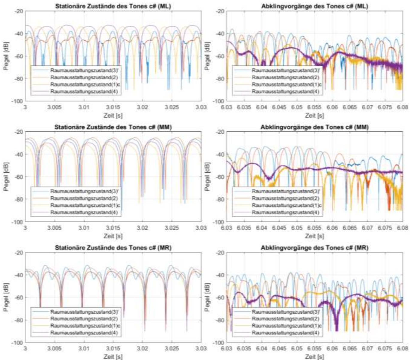
Abb. B2.14: Messsignalwellenformen der Marimbatonmessungen bei Anregung von Quellposition (Q2) mit der Grundfrequenz des Tones c# ( \approx 140 Hz) für alle vier Raumausstattungszustände (3)j, (2), (1)c und (4) sowie die Mikrofonpositionen (ML), (MM) und (MR)
