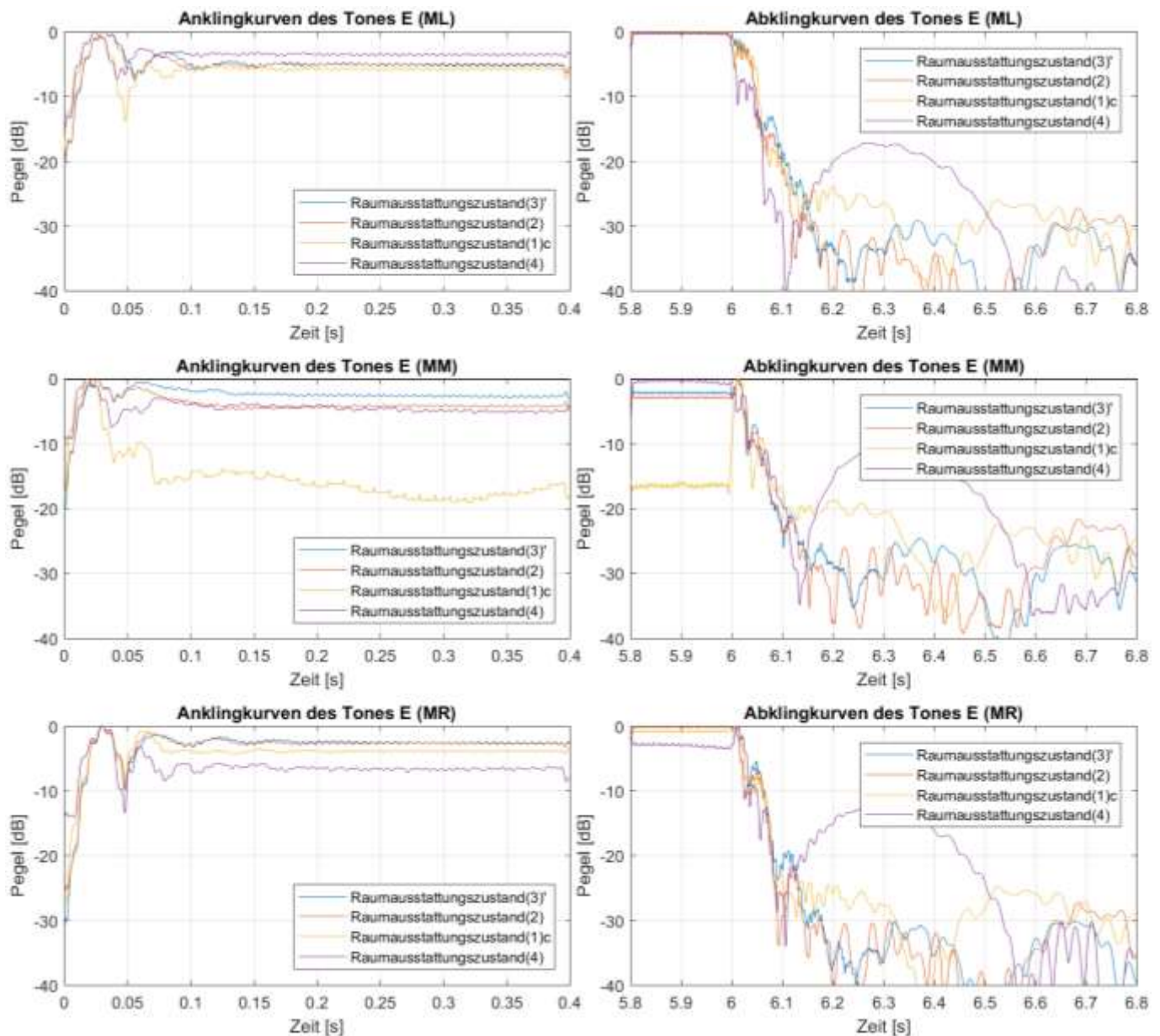
Abb. 6.20: An- und Abklingkurven der Marimbatonmessungen bei Anregung von Quellposition (Q1) mit der Grundfrequenz des Tones E ( \cong 83 Hz) für alle vier Raumausstattungs Zustände (3)', (2), (1)c und (4) sowie die Mikrofonpositionen (ML), (MM) und (MR)
