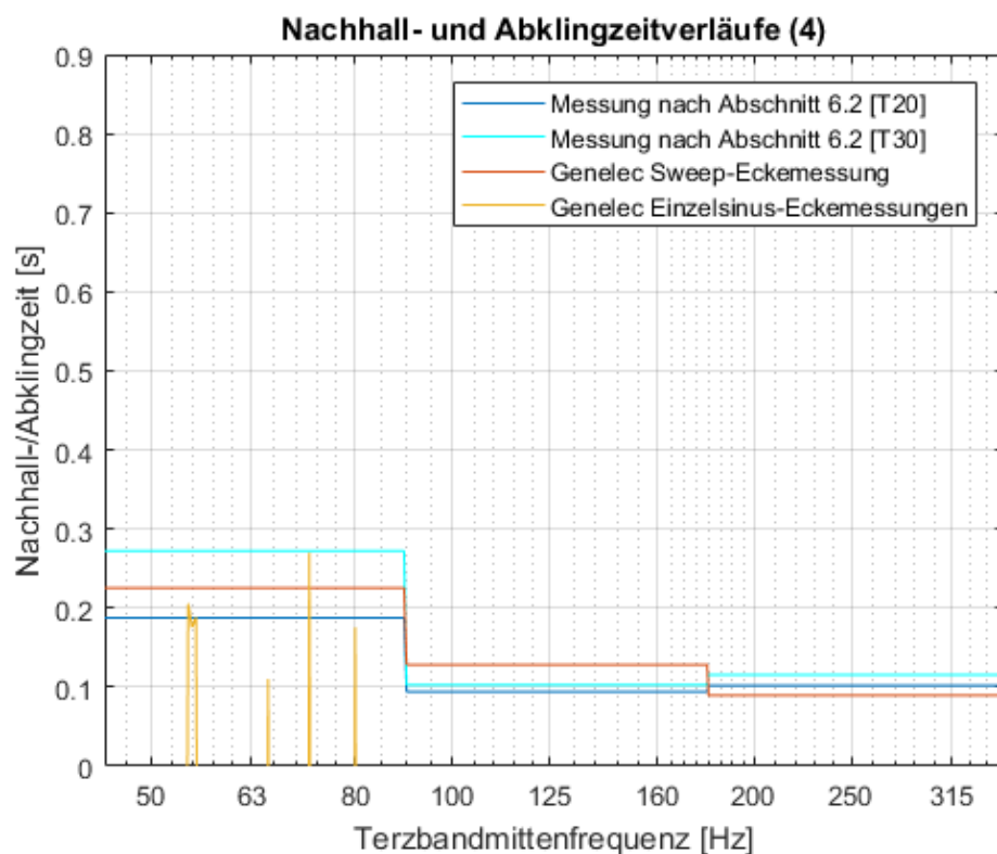
Abb. 6.14: Nachhall- und Einzelsinusabklingzeitverläufe bei „Eckmessungen“ mit dem Genelec Studiomonitor zum Raumausstattungszustand (4) mit Hinterlegung des Nachhallzeitverlaufs aus Abschnitt 6.2
