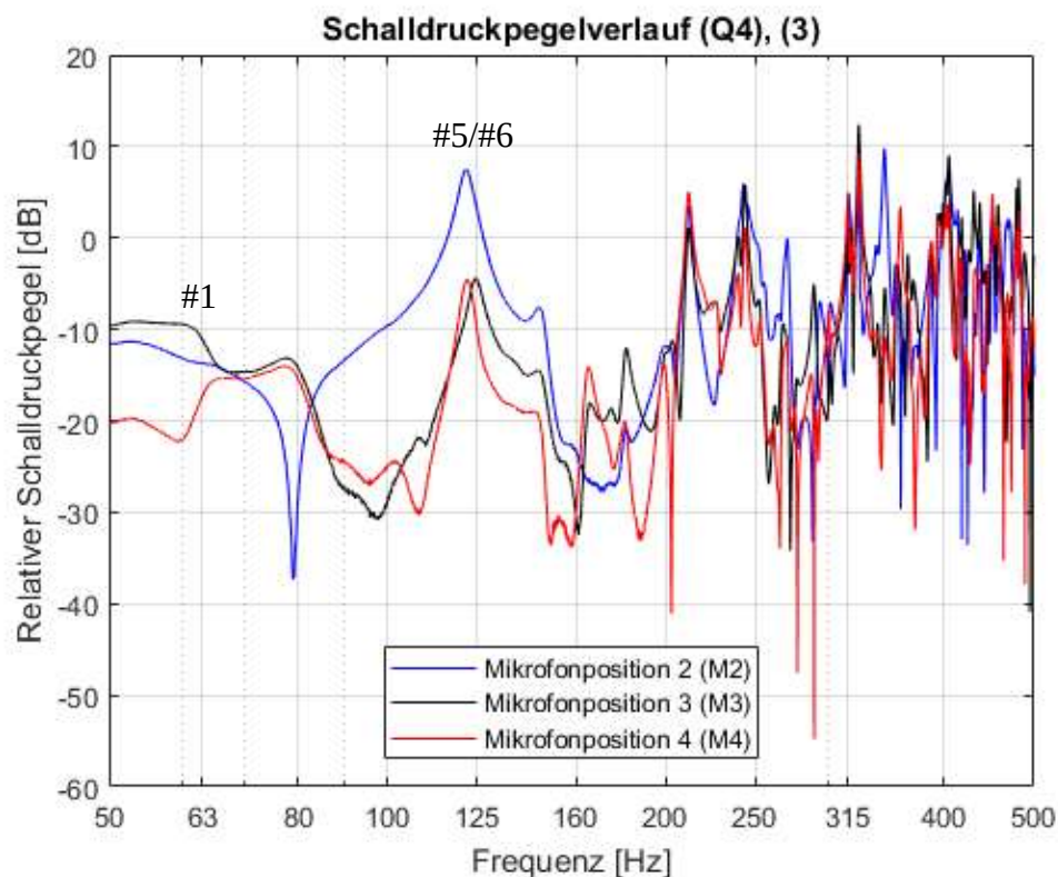
Abb. 5.21: Relative Schalldruckpegelverläufe für den mittleren Marimbatonbereich (Q4) zum Zustand (3) an der Hauptspielerposition (M2) sowie der linksten (M3) und rechten (M4) Spielerposition
