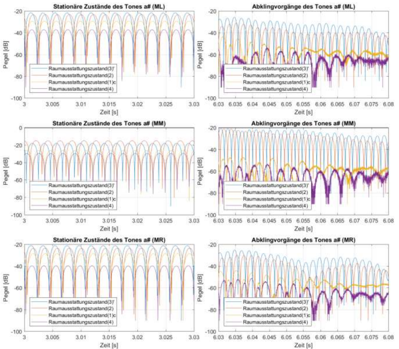
Abb. B2.23: Messsignalwellenformen der Marimbatonmessungen bei Anregung von Quellposition (Q3) mit der Grundfrequenz des Tones a# ( \cong 235 Hz) für alle vier Raumausstattungs Zustände (3)', (2), (1)c und (4) sowie die Mikrofonpositionen (ML), (MM) und (MR)
