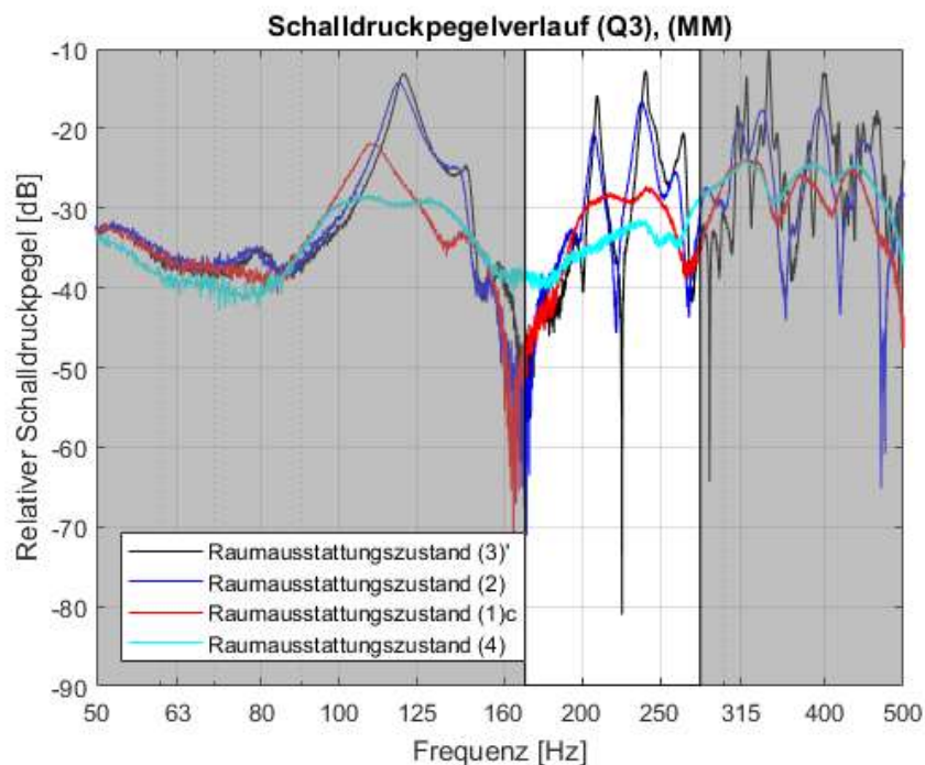
Abb. 6.28: Relative Schalldruckpegelverläufe für den tiefmittleren Marimbatonbereich f-c# ( Q3 ) zu den vier verschiedenen Raumausstattungs Zuständen ( 3) ', ( 2 ), ( 1 )c und ( 4 ) an der Hauptspielerposition ( MM )
