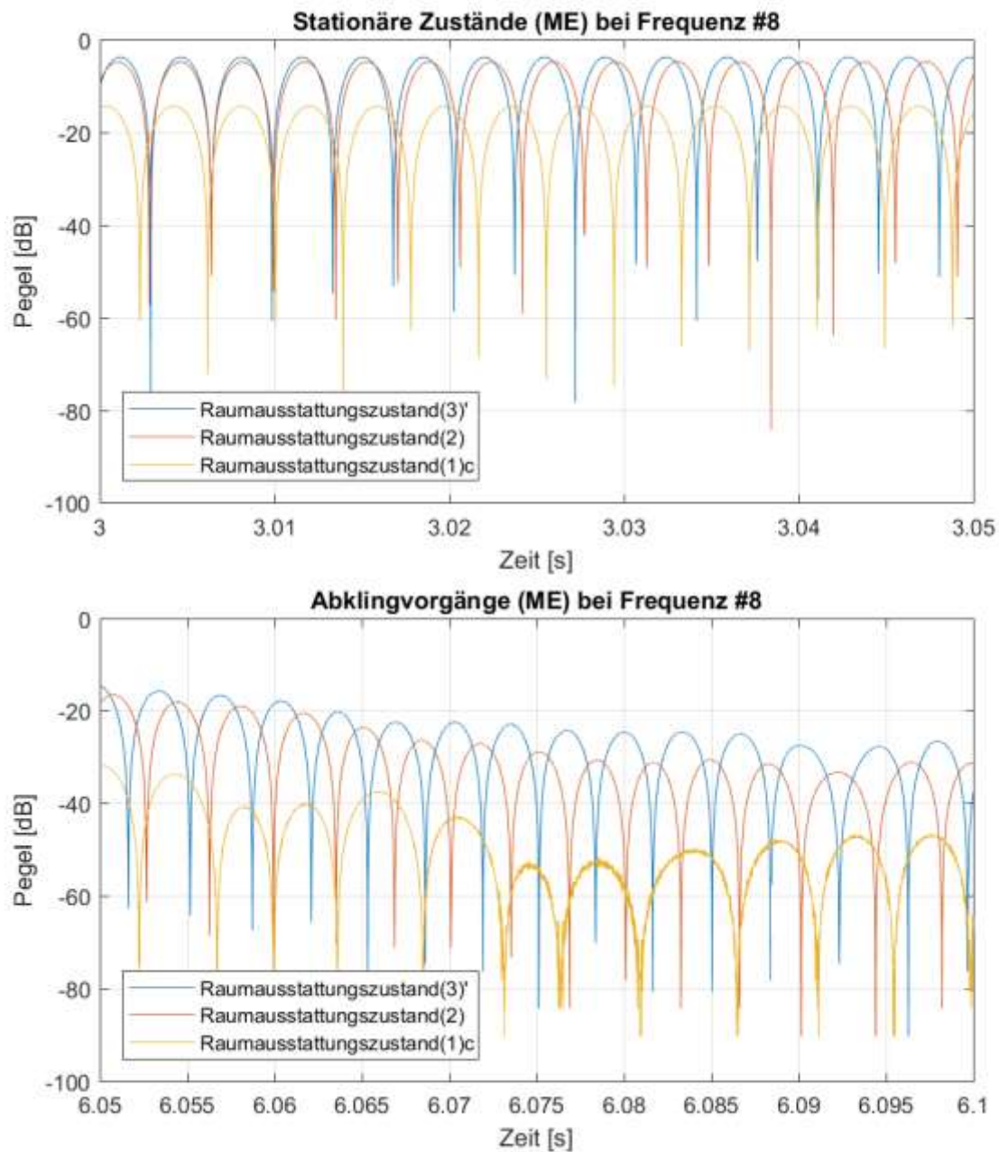
Abb. A2.8: Messsignalwellenformen der Eckmessungen bei Anregung mit Frequenz #8 für die drei Raumausstattungsstände (3)', (2) und (1)c
