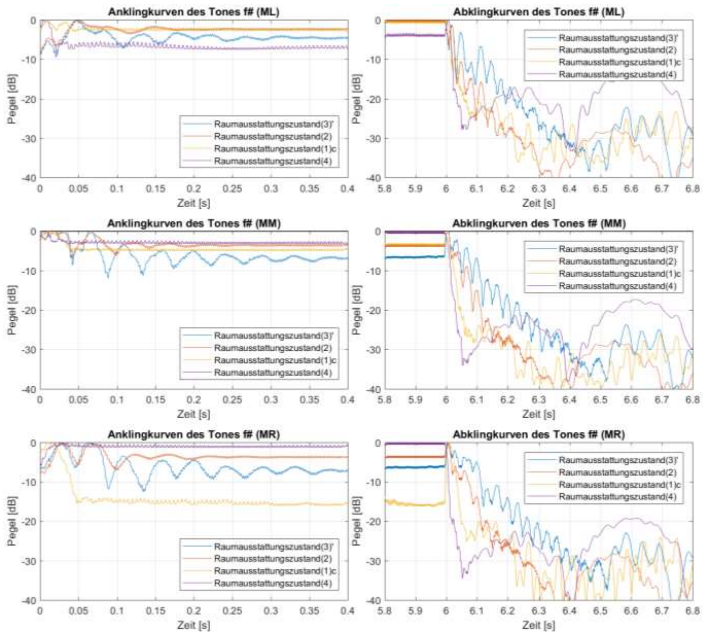
Abb. B1.19: An- und Abklingkurven der Marimbatonmessungen bei Anregung von Quellposition ( Q3 ) mit der Grundfrequenz des Tones f# ( \cong 186 Hz) für alle vier Raumausstattungszustände ( 3' , 2 ), (1)c und 4 ) sowie die Mikrofonpositionen ( ML ), ( MM ) und ( MR )
