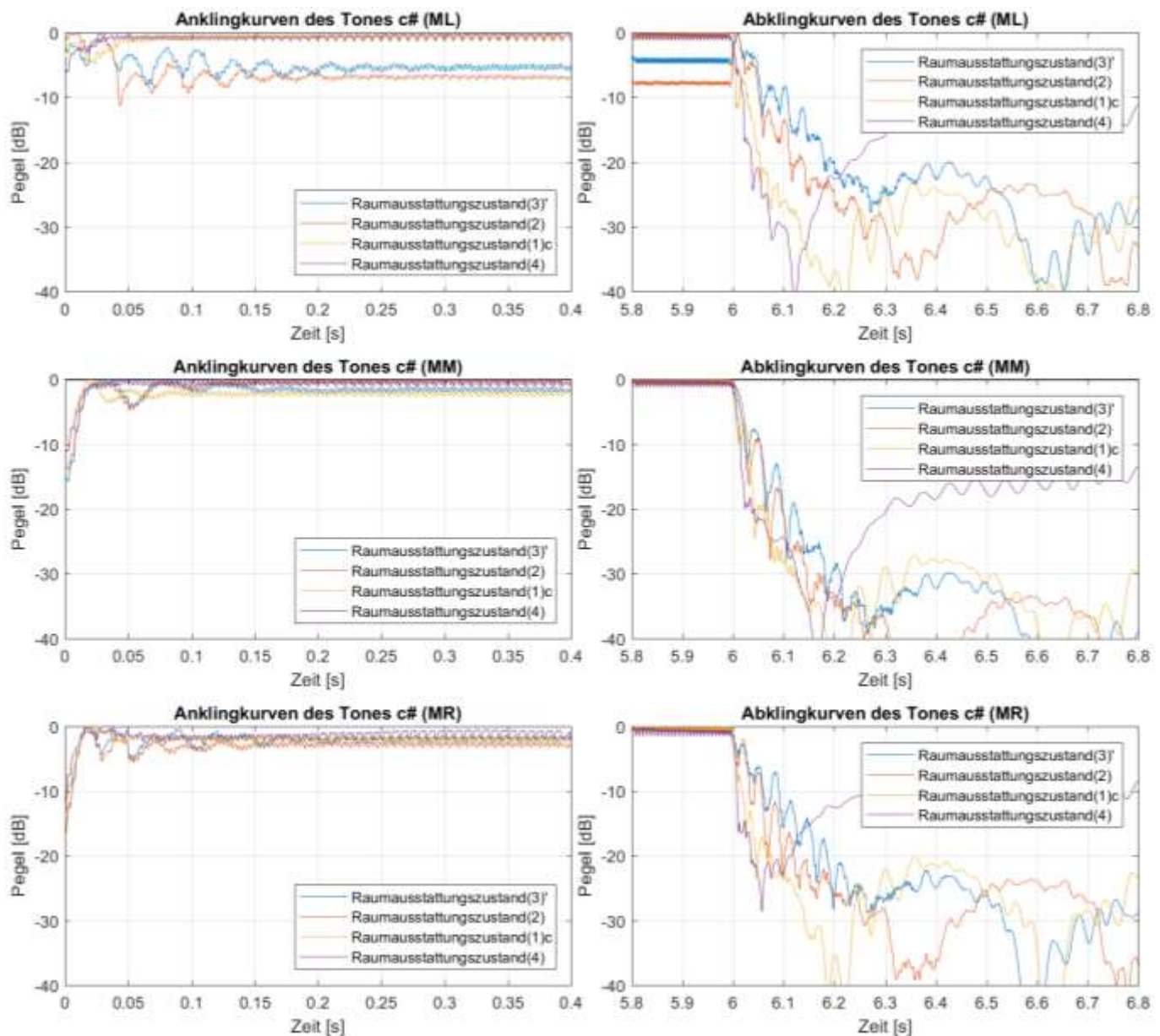
Abb. B1.14: An- und Abklingkurven der Marimbatonmessungen bei Anregung von Quellposition (Q2) mit der Grundfrequenz des Tones c# ( \triangleq 140 Hz) für alle vier Raumausstattungs Zustände (3)', (2), (1)c und (4) sowie die Mikrofonpositionen (ML), (MM) und (MR)
