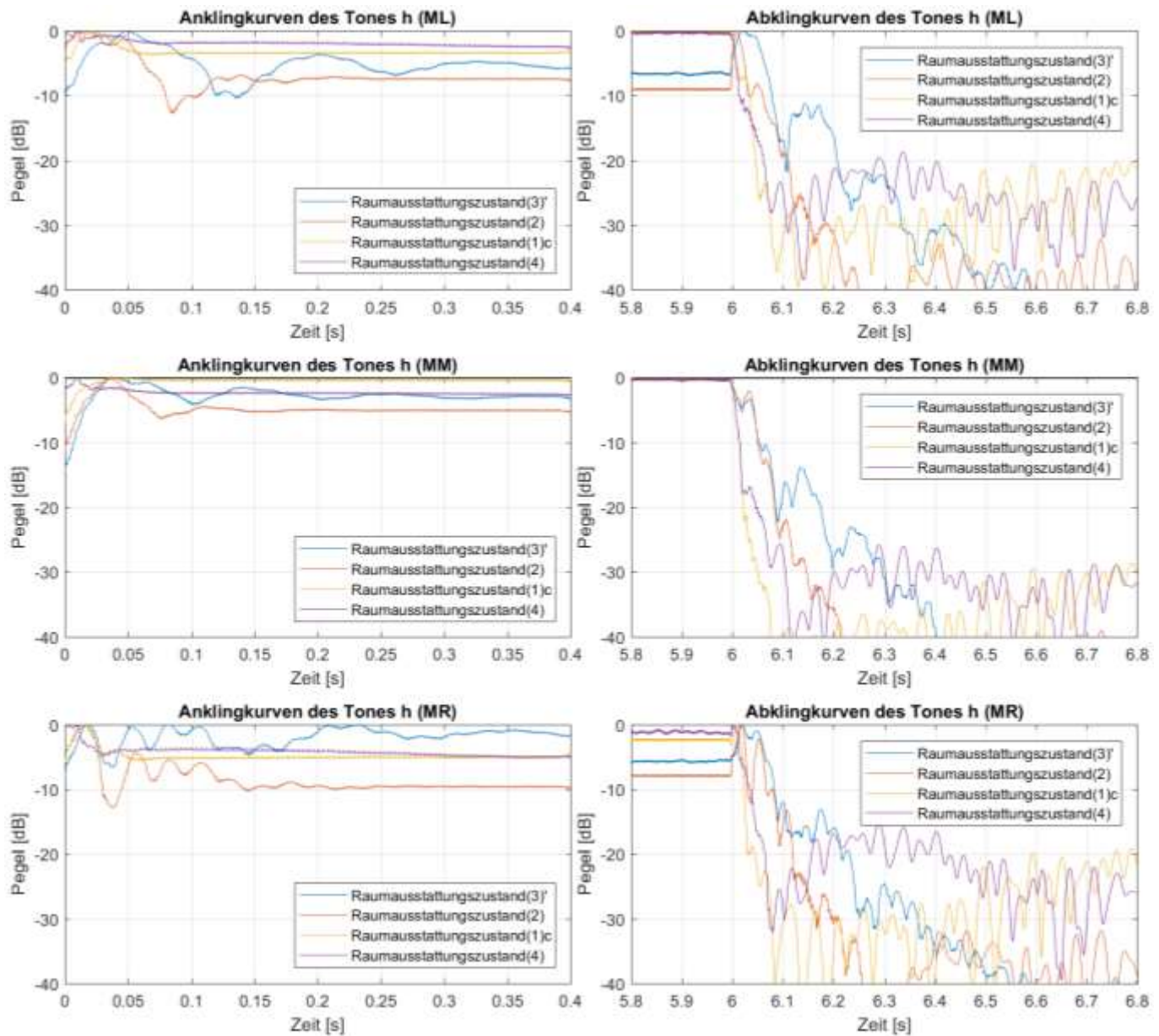
Abb. B1.24: An- und Abklingkurven der Marimbatonmessungen bei Anregung von Quellposition ( Q3 ) mit der Grundfrequenz des Tones h ( \cong 249 Hz) für alle vier Raumausstattungs Zustände ( 3' , (2) , (1)c und (4) sowie die Mikrofonpositionen ( ML ), ( MM ) und ( MR )
