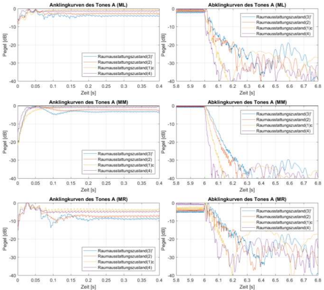
Abb. B1.10: An- und Abklingkurven der Marimbatonmessungen bei Anregung von Quellposition ( Q2 ) mit der Grundfrequenz des Tones A ( \cong 111 Hz) für alle vier Raumausstattungszustände ( 3' , (2) , (1)c und (4) sowie die Mikrofonpositionen ( ML ), ( MM ) und ( MR )
