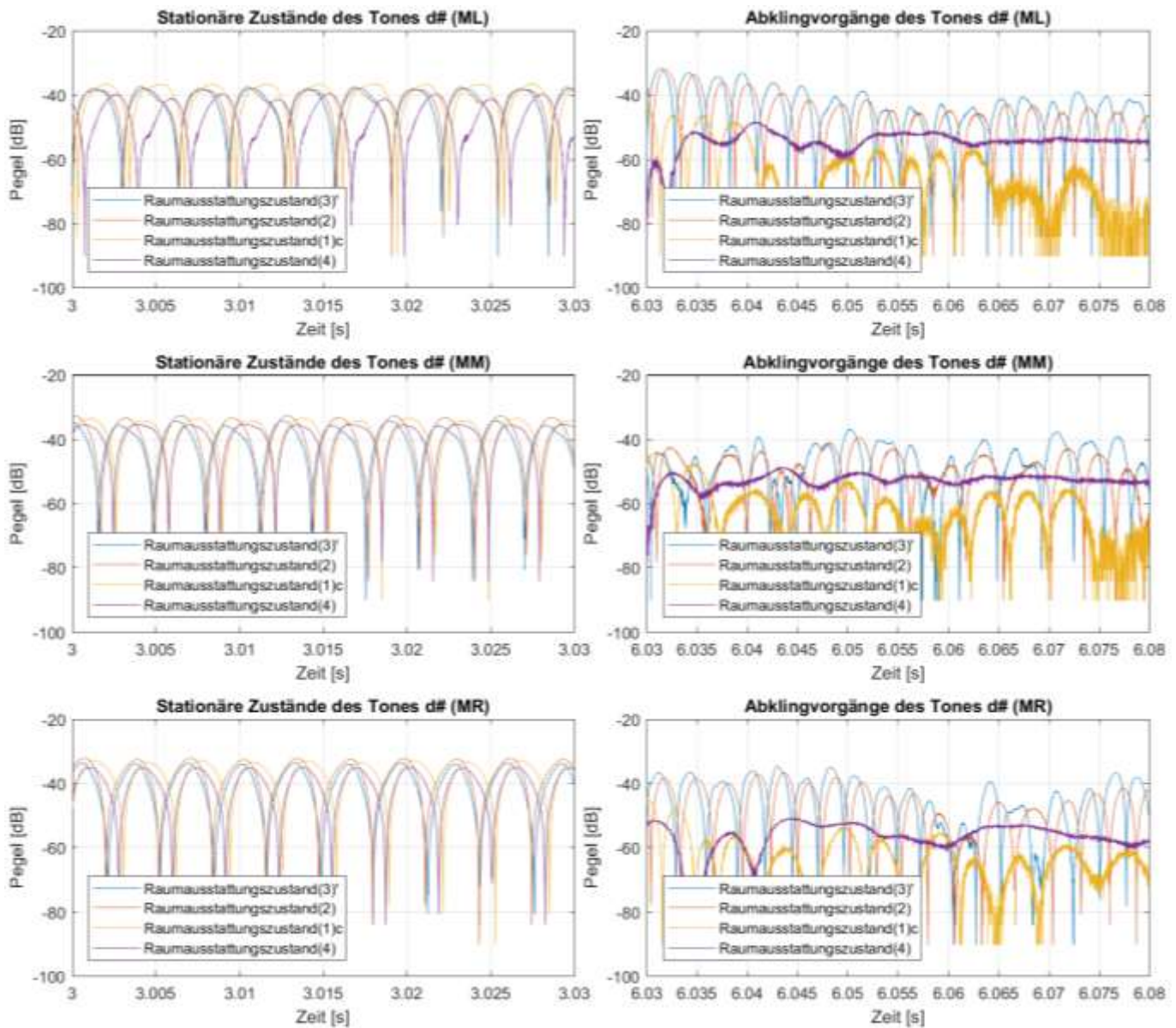
Abb. B2.16: Messsignalwellenformen der Marimbatonmessungen bei Anregung von Quellposition (Q2) mit der Grundfrequenz des Tones d# ( \cong 157 Hz) für alle vier Raumausstattungs Zustände (3) f , (2), (1)c und (4) sowie die Mikrofonpositionen (ML), (MM) und (MR)
