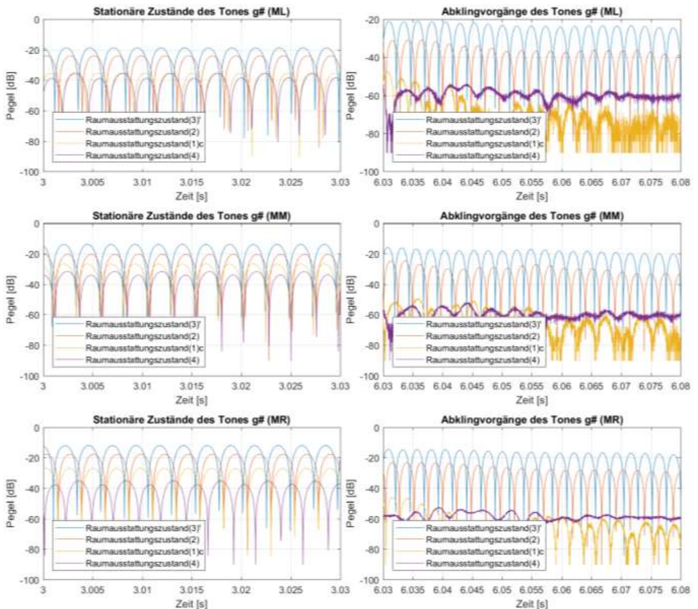
Abb. B2.21: Messsignalwellenformen der Marimbatonmessungen bei Anregung von Quellposition (Q3) mit der Grundfrequenz des Tones g# ( \cong 209 Hz) für alle vier Raumausstattungs Zustände (3) f , (2), (1) c und (4) sowie die Mikrofonpositionen (ML), (MM) und (MR)
