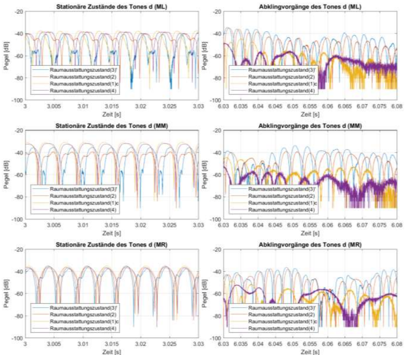
Abb. B2.15: Messsignalwellenformen der Marimbatonmessungen bei Anregung von Quellposition (Q2) mit der Grundfrequenz des Tones d ( \cong 148 Hz) für alle vier Raumausstattungs Zustände (3)', (2), (1)c und (4) sowie die Mikrofonpositionen (ML), (MM) und (MR)
