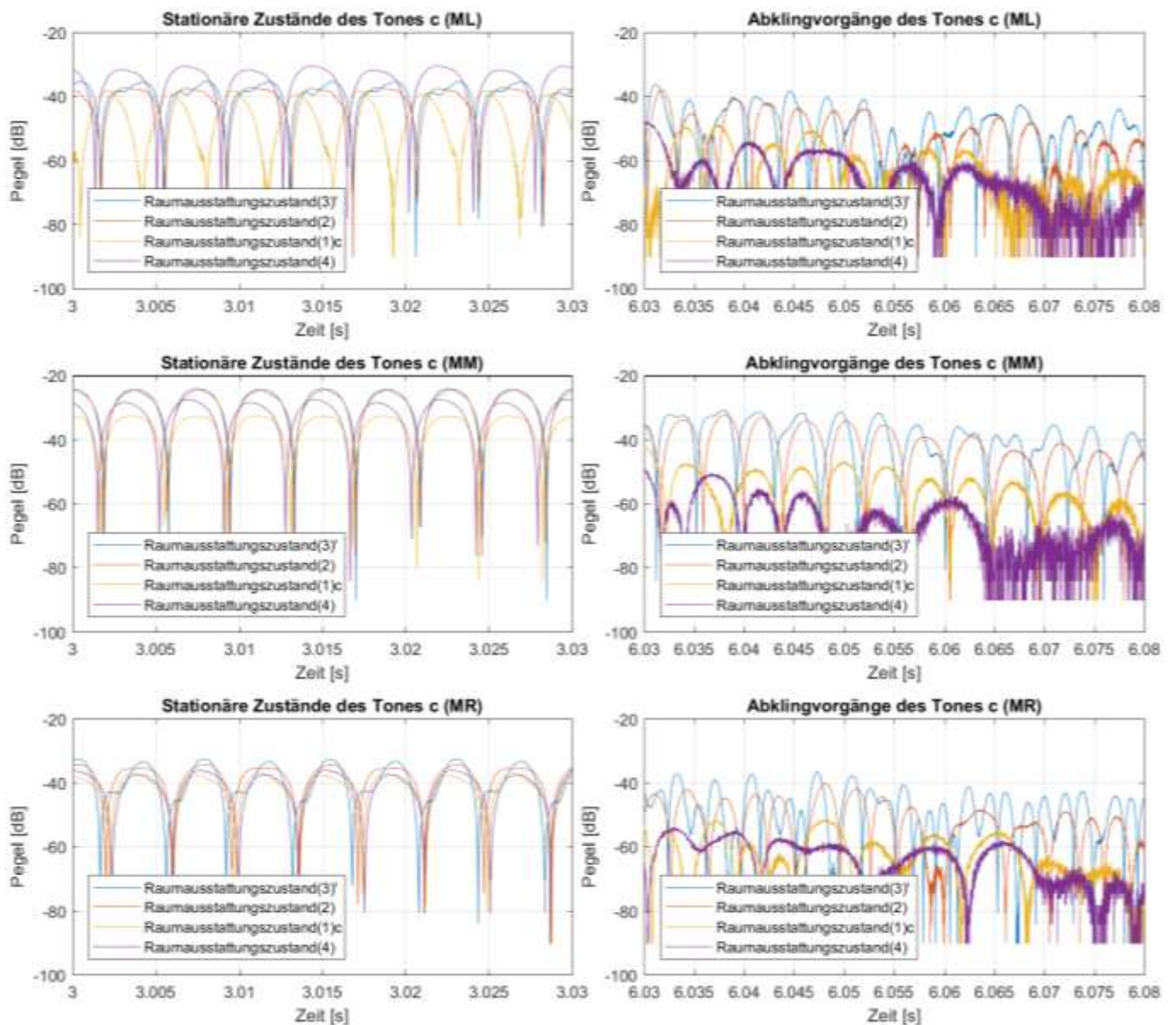
Abb. B2.13: Messsignalwellenformen der Marimbatonmessungen bei Anregung von Quellposition (Q2) mit der Grundfrequenz des Tones c ( \approx 132 Hz) für alle vier Raumausstattungs Zustände (3) f , (2), (1)c und (4) sowie die Mikrofonpositionen (ML), (MM) und (MR)
