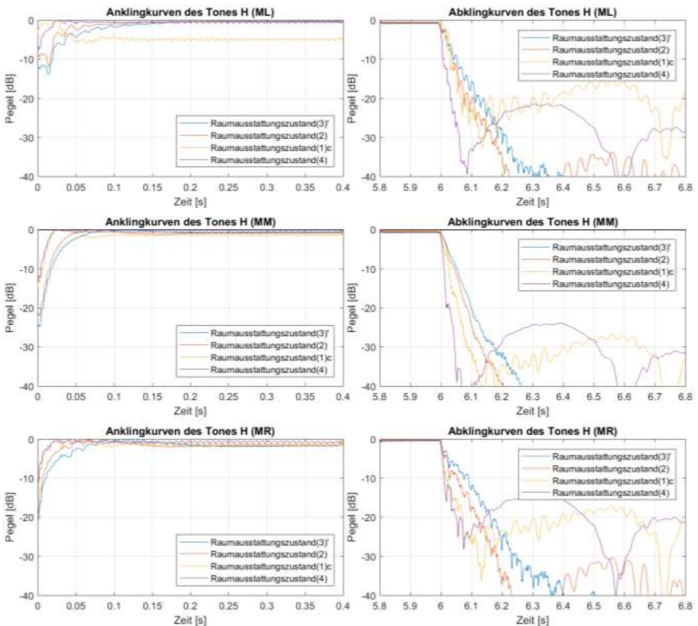
Abb. 6.21: An- und Abklingkurven der Marimbatonmessungen bei Anregung von Quellposition (Q2) mit der Grundfrequenz des Tones H ( \cong 124 Hz) für alle vier Raumausstattungszustände (3)', (2), (1)c und (4) sowie die Mikrofonpositionen (ML), (MM) und (MR)
