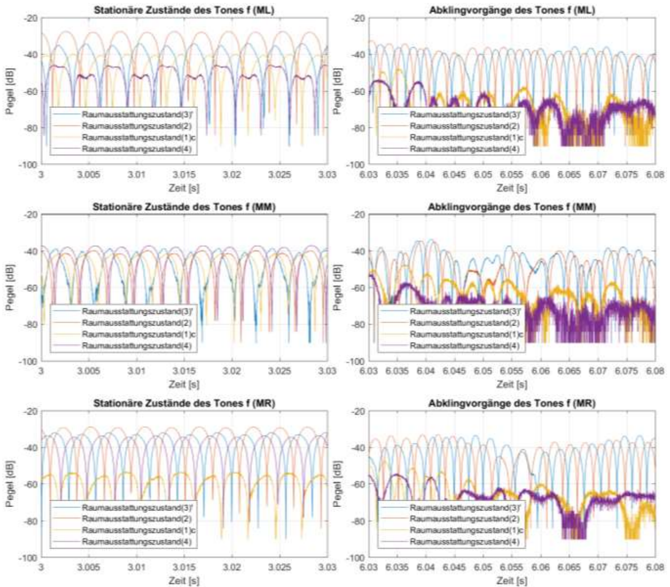
Abb. B2.18: Messsignalwellenformen der Marimbatonmessungen bei Anregung von Quellposition (Q3) mit der Grundfrequenz des Tones f ( \cong 176 Hz) für alle vier Raumausstattungs Zustände (3) * , (2), (1)c und (4) sowie die Mikrofonpositionen (ML), (MM) und (MR)
