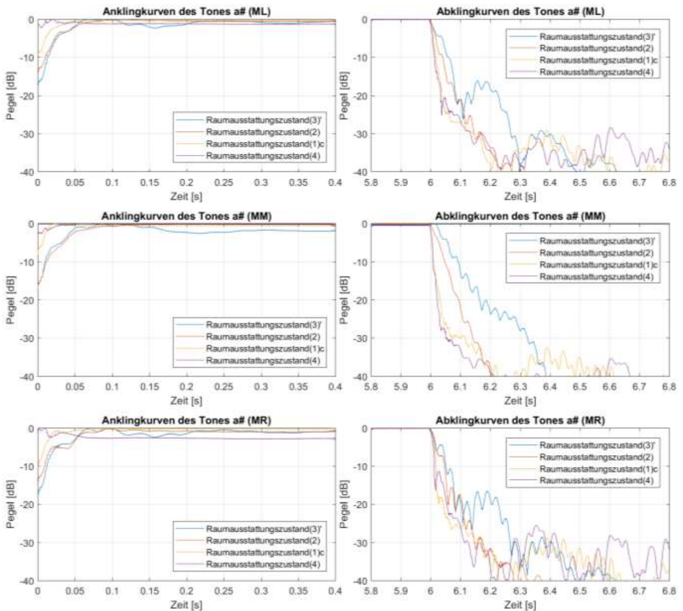
Abb. B1.23: An- und Abklingkurven der Marimbatonmessungen bei Anregung von Quellposition ( Q3 ) mit der Grundfrequenz des Tones a# ( \cong 235 Hz) für alle vier Raumausstattungs Zustände ( 3 ), ( 2 ), ( 1 )c und ( 4 ) sowie die Mikrofonpositionen ( ML ), ( MM ) und ( MR )
