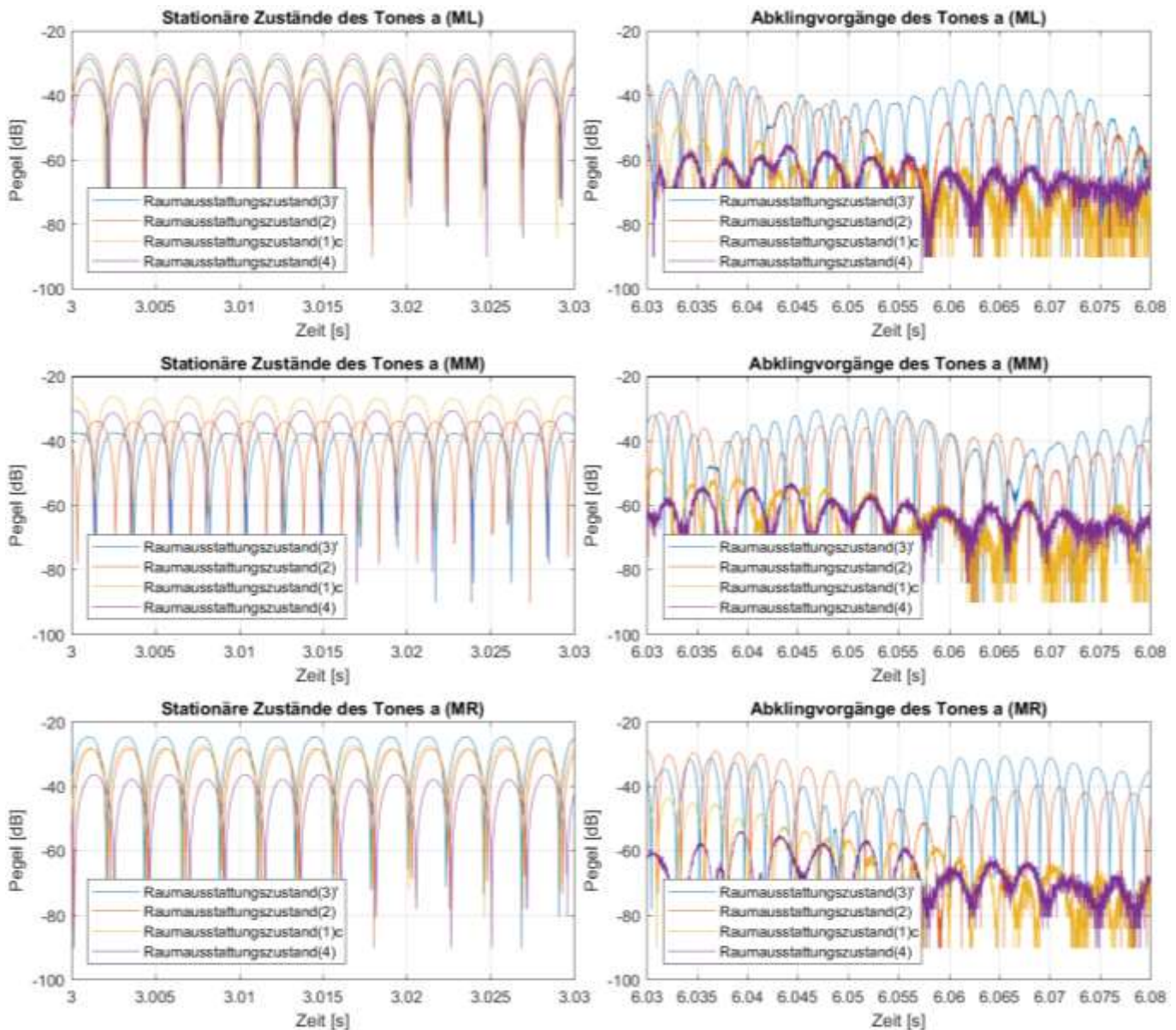
Abb. B2.22: Messsignalwellenformen der Marimbatonmessungen bei Anregung von Quellposition (Q3) mit der Grundfrequenz des Tones a ( \approx 222 Hz) für alle vier Raumausstattungszustände (3) + , (2), (1)c und (4) sowie die Mikrofonpositionen (ML), (MM) und (MR)
