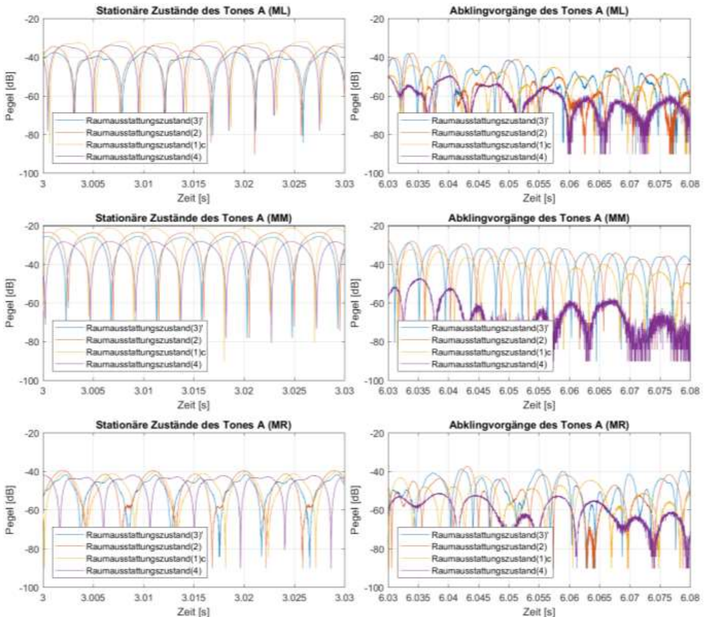
Abb. B2.10: Messsignalwellenformen der Marimbatonmessungen bei Anregung von Quellposition (Q2) mit der Grundfrequenz des Tones A ( \cong 111 Hz) für alle vier Raumausstattungs Zustände (3) f , (2), (1) c und (4) sowie die Mikrofonpositionen (ML), (MM) und (MR)
