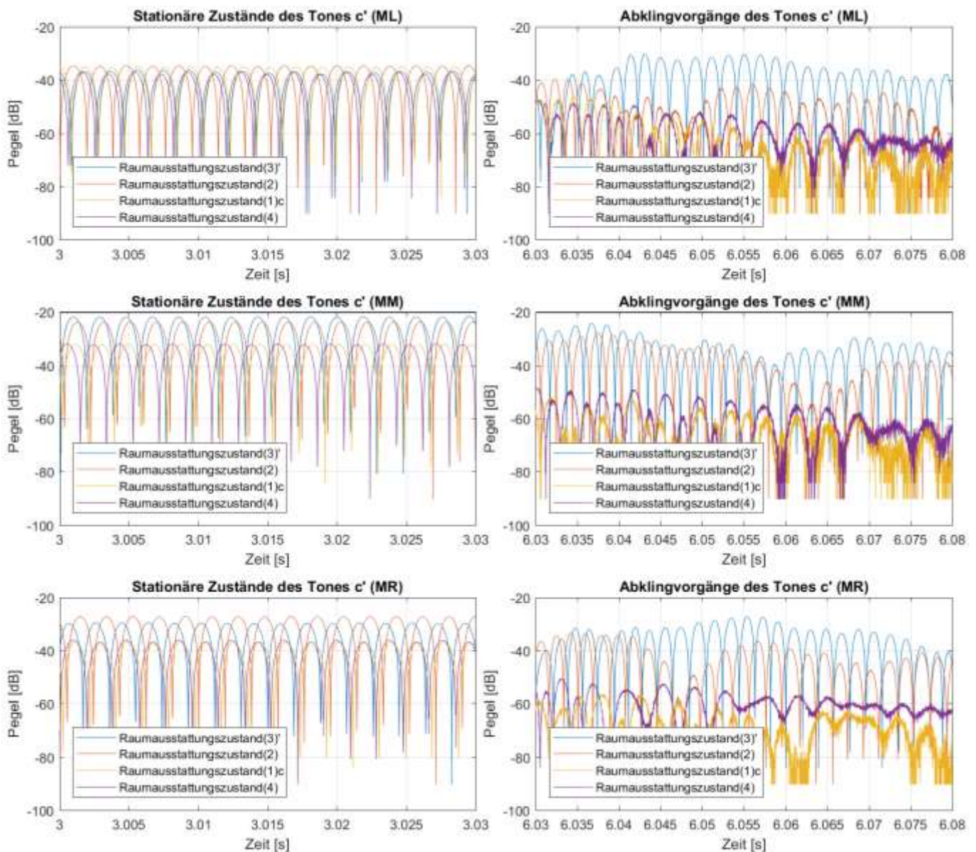
Abb. B2.25: Messsignalwellenformen der Marimbatonmessungen bei Anregung von Quellposition (Q3) mit der Grundfrequenz des Tones c' ( \approx 263 Hz) für alle vier Raumausstattungs Zustände (3)', (2), (1)c und (4) sowie die Mikrofonpositionen (ML), (MM) und (MR)
