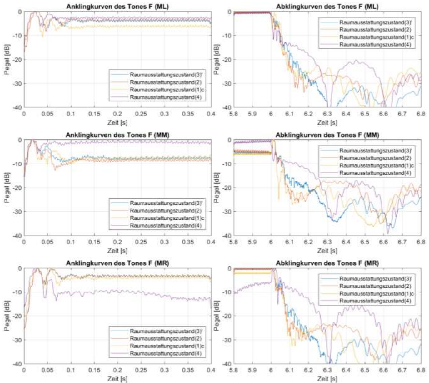
Abb. B1.6: An- und Abklingkurven der Marimbatonmessungen bei Anregung von Quellposition ( Q1 ) mit der Grundfrequenz des Tones F ( \triangleq 88 Hz) für alle vier Raumausstattungs Zustände ( 3 )', ( 2 ), ( 1 )c und ( 4 ) sowie die Mikrofonpositionen ( ML ), ( MM ) und ( MR )
