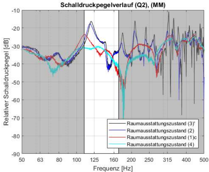
Abb. 6.27: Relative Schalldruckpegelverläufe für den mitteltiefen Marimbatonbereich A-e ( Q2 ) zu den vier verschiedenen Raumausstattungs Zuständen ( 3) ', ( 2 ), ( 1 )c und ( 4 ) an der Hauptspielerposition ( MM )
