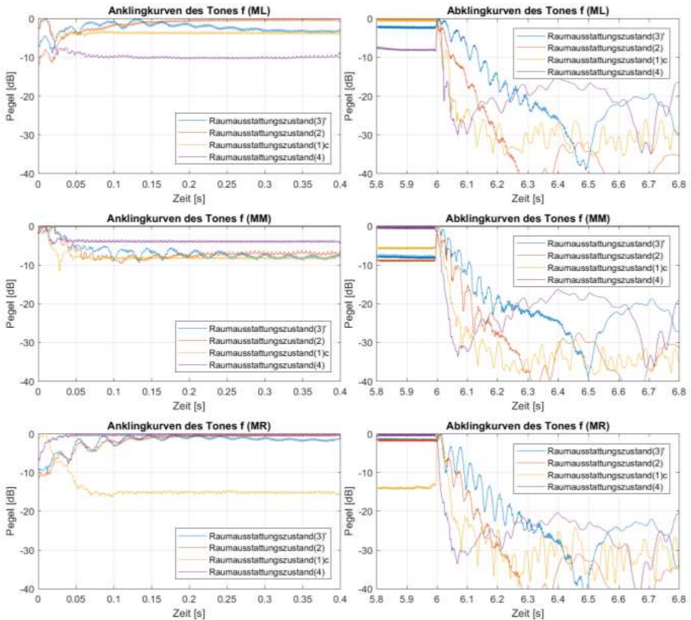
Abb. B1.18: An- und Abklingkurven der Marimbatonmessungen bei Anregung von Quellposition (Q3) mit der Grundfrequenz des Tones f ( \cong 176 Hz) für alle vier Raumausstattungs Zustände (3)', (2), (1)c und (4) sowie die Mikrofonpositionen (ML), (MM) und (MR)
