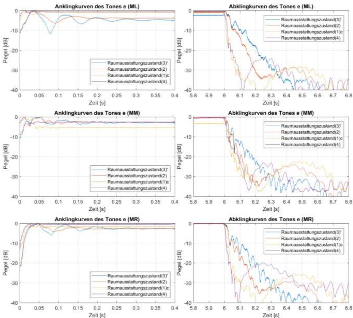
Abb. B1.17: An- und Abklingkurven der Marimbatonmessungen bei Anregung von Quellposition ( Q2 ) mit der Grundfrequenz des Tones e ( \cong 166 Hz) für alle vier Raumausstattungs Zustände ( 3' ), ( 2 ), ( 1 )c und ( 4 ) sowie die Mikrofonpositionen ( ML ), ( MM ) und ( MR )
