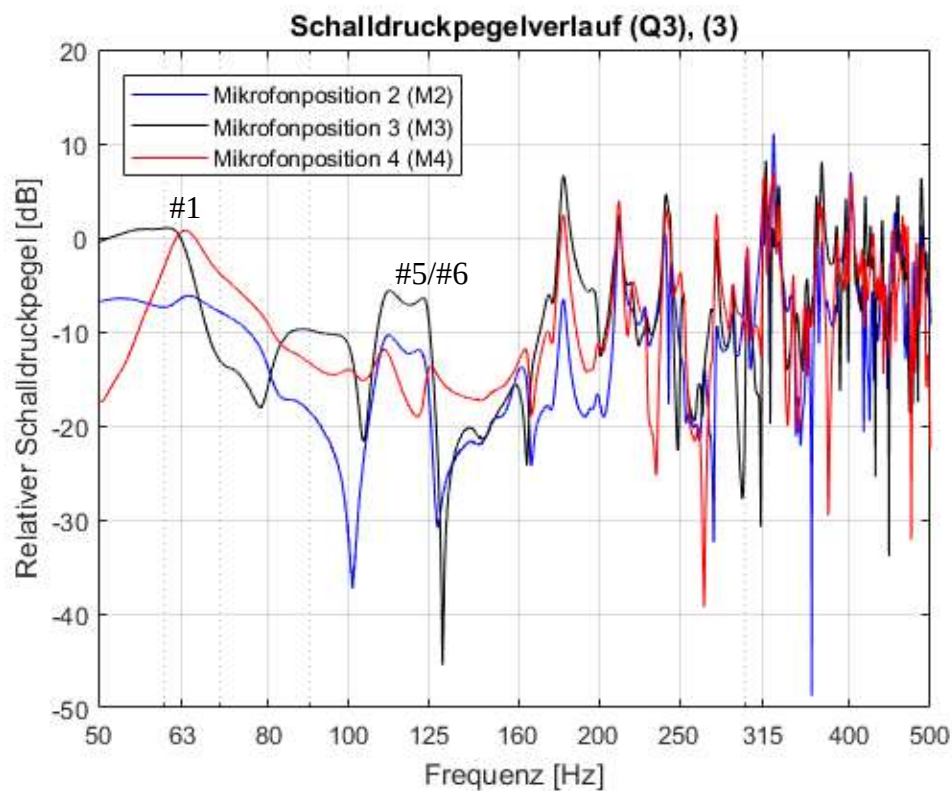
Abb. 5.22: Relative Schalldruckpegelverläufe für den hohen Marimbatonbereich (Q3) zum Zustand (3) an der Hauptspielerposition (M2) sowie der linksten (M3) und rechten (M4) Spielerposition
