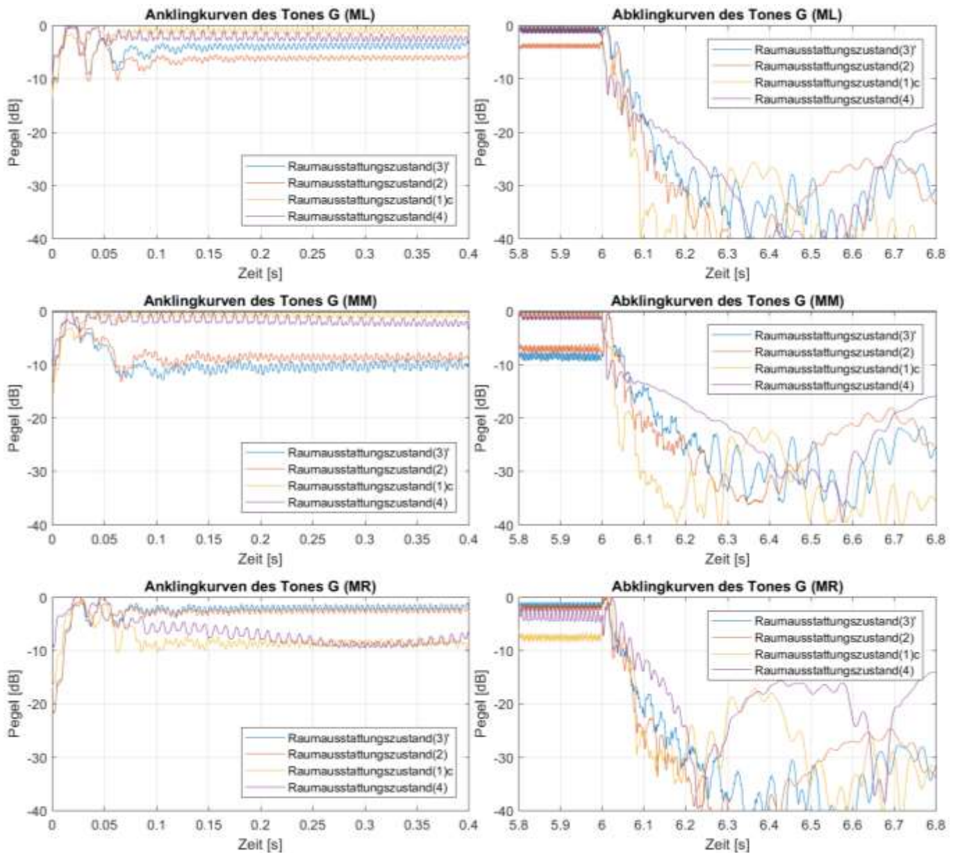
Abb. B1.8: An- und Abklingkurven der Marimbatonmessungen bei Anregung von Quellposition ( Q1 ) mit der Grundfrequenz des Tones G ( \cong 99 Hz) für alle vier Raumausstattungs Zustände ( (3)' , (2) , (1)c und (4) sowie die Mikrofonpositionen ( (ML) , (MM) und (MR) )
