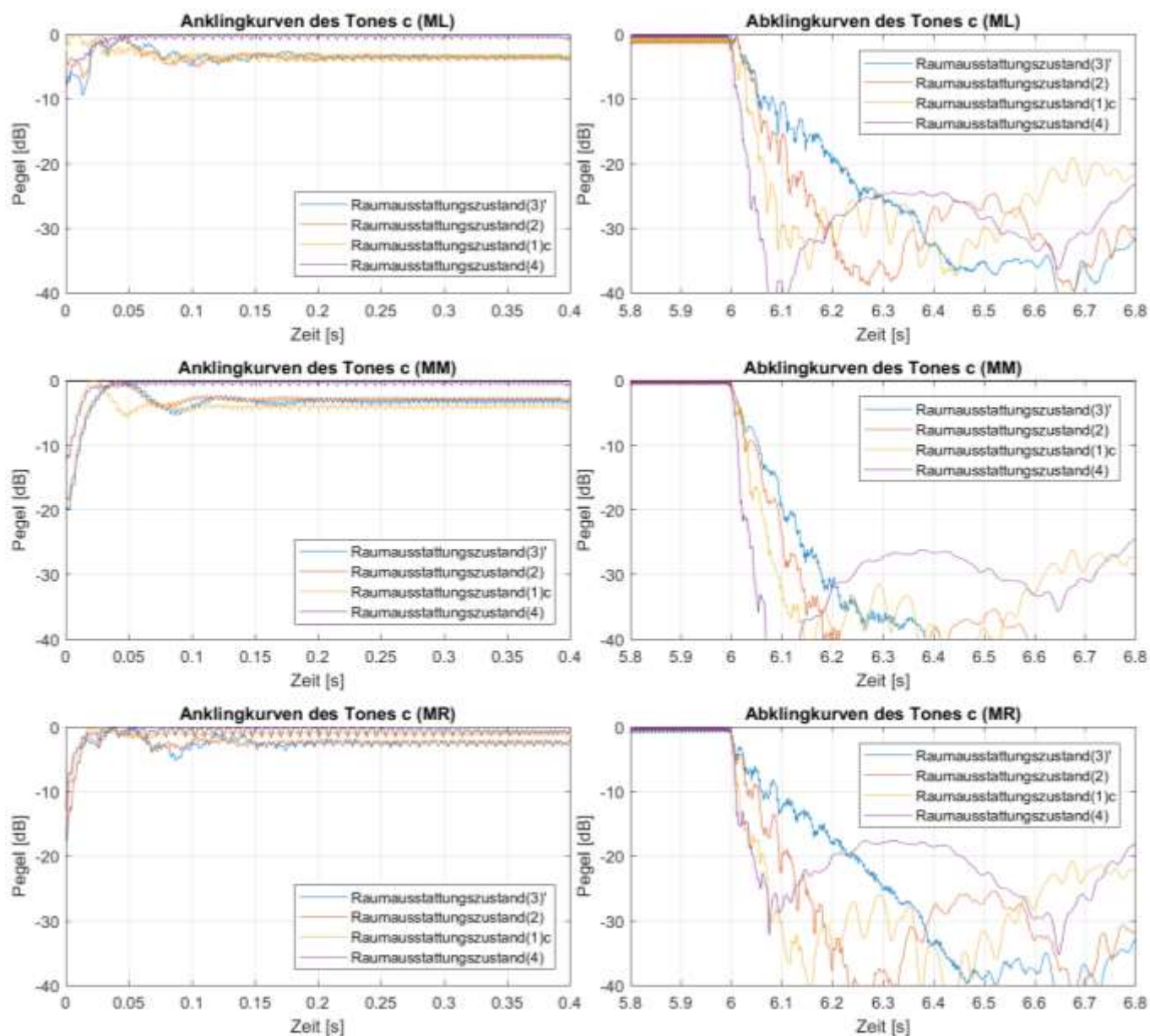
Abb. B1.13: An- und Abklingkurven der Marimbatonmessungen bei Anregung von Quellposition ( Q2 ) mit der Grundfrequenz des Tones c ( \cong 132 Hz) für alle vier Raumausstattungs Zustände ( 3' ), ( 2 ), ( 1 )c und ( 4 ) sowie die Mikrofonpositionen ( ML ), ( MM ) und ( MR )
