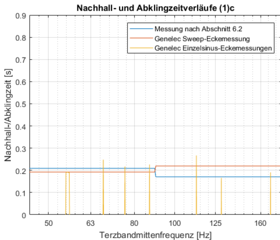
Abb. 6.13: Nachhall- und Einzelsinusabklingzeitverläufe bei „Eckmessungen“ mit dem Genelec Studiomonitor zum Raumausstattungszustand (1)c mit Hinterlegung des Nachhallzeitverlaufs aus Abschnitt 6.2
