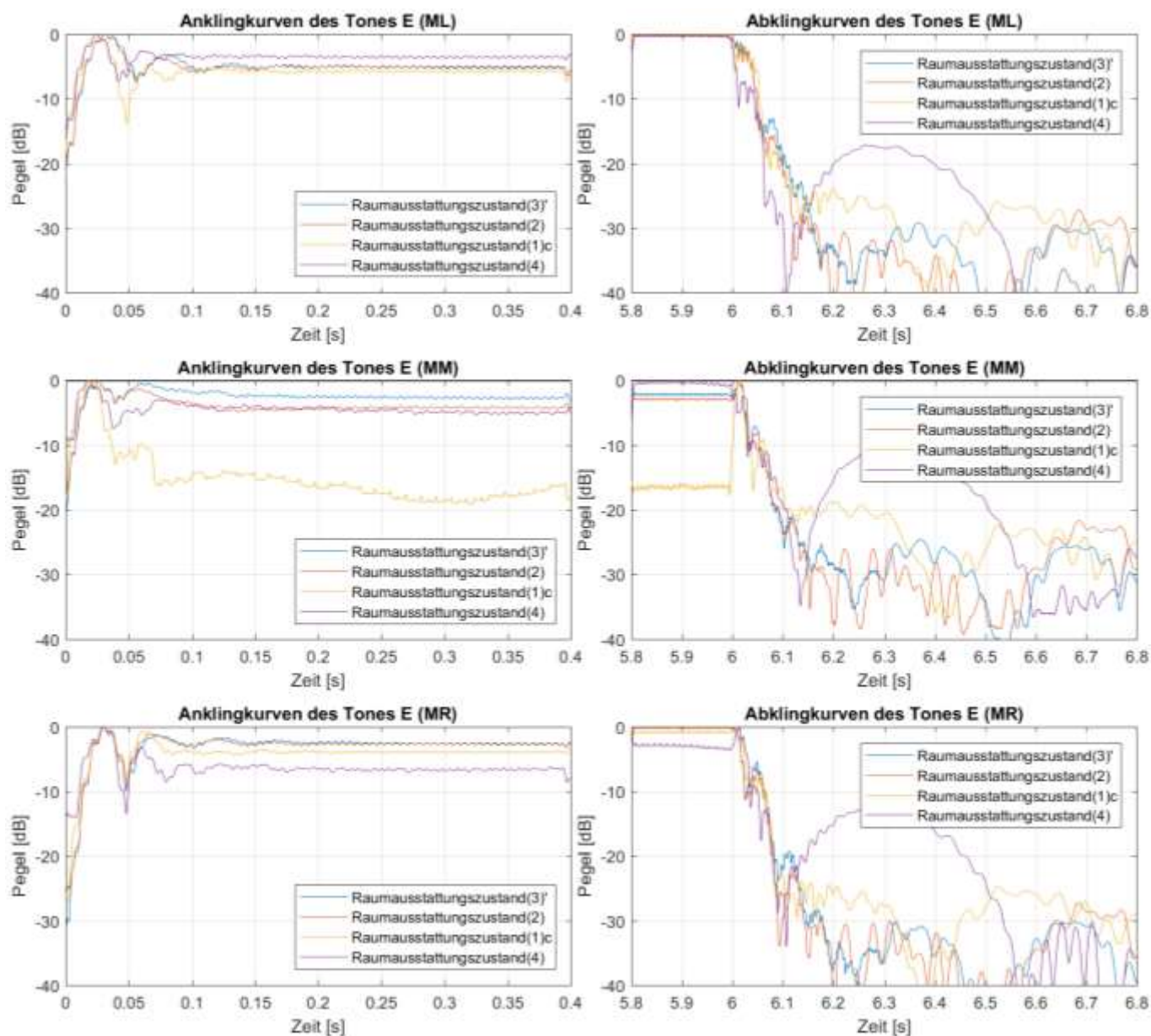
Abb. B1.5: An- und Abklingkurven der Marimbatonmessungen bei Anregung von Quellposition ( Q1 ) mit der Grundfrequenz des Tones E ( \cong 83 Hz) für alle vier Raumausstattungs Zustände ( (3)' , (2) , (1)c und (4) sowie die Mikrofonpositionen ( ML ), ( MM ) und ( MR )
