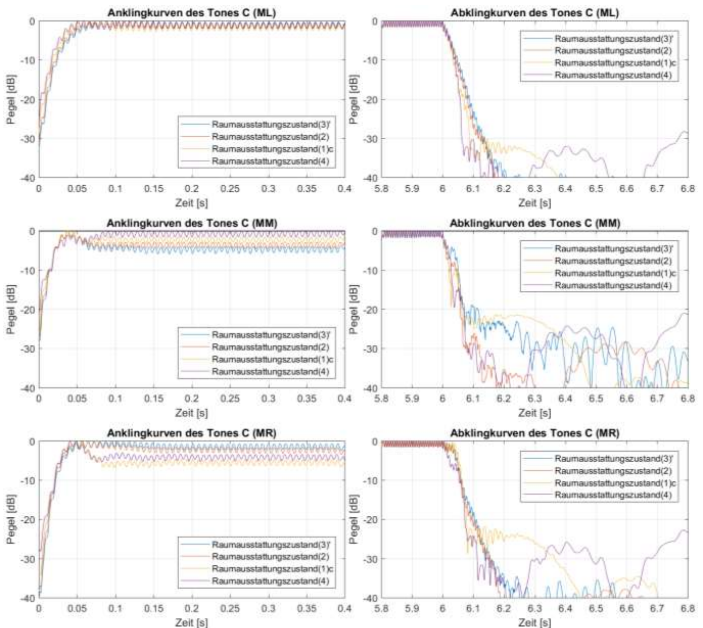
Abb. B1.1: An- und Abklingkurven der Marimbatonmessungen bei Anregung von Quellposition (Q1) mit der Grundfrequenz des Tones C ( \cong 66 Hz) für alle vier Raumausstattungs Zustände (3)', (2), (1)c und (4) sowie die Mikrofonpositionen (ML), (MM) und (MR)
