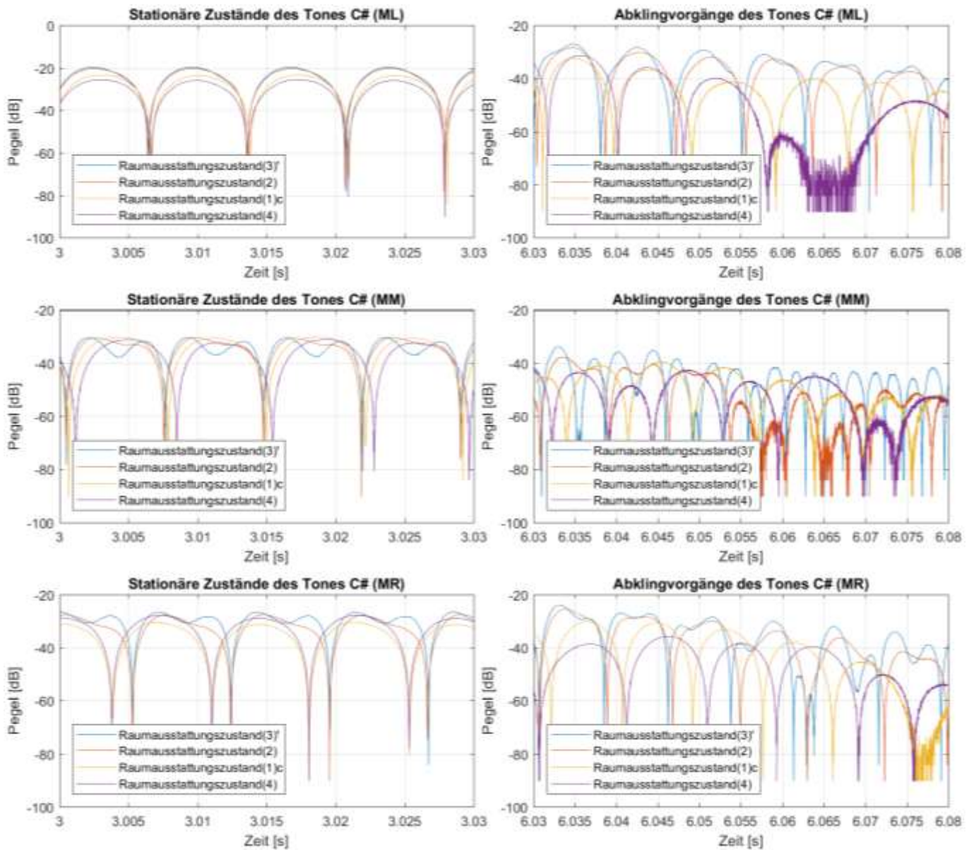
Abb. B2.2: Messsignalwellenformen der Marimbatonmessungen bei Anregung von Quellposition (Q1) mit der Grundfrequenz des Tones C# ( \cong 70 Hz) für alle vier Raumausstattungs Zustände (3) f , (2), (1)c und (4) sowie die Mikrofonpositionen (ML), (MM) und (MR)
