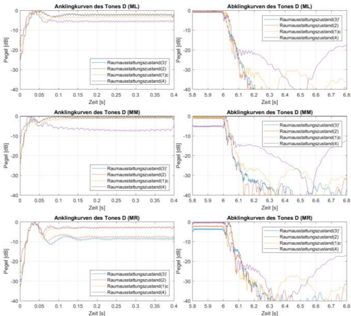
Abb. B1.3: An- und Abklingkurven der Marimbatonmessungen bei Anregung von Quellposition ( Q1 ) mit der Grundfrequenz des Tones D ( \cong 74 Hz) für alle vier Raumausstattungs Zustände ( 3' , (2) , (1)c und (4) sowie die Mikrofonpositionen ( ML ), ( MM ) und ( MR )
