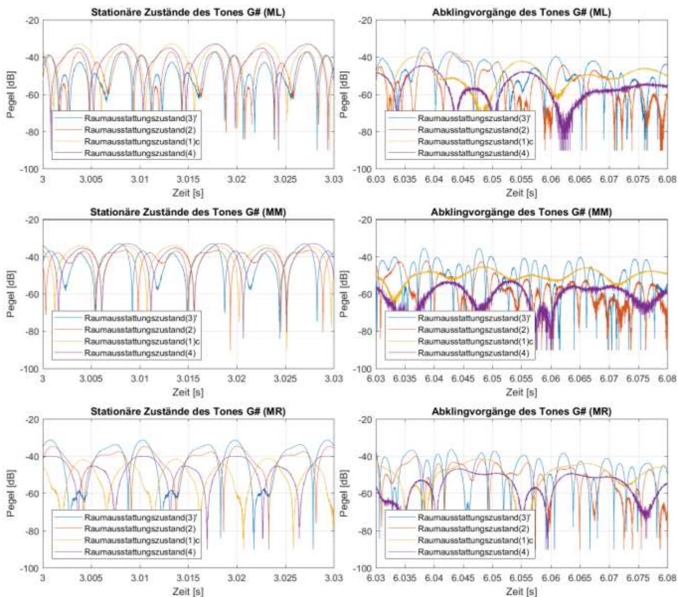
Abb. B2.9: Messsignalwellenformen der Marimbatonmessungen bei Anregung von Quellposition ( Q1 ) mit der Grundfrequenz des Tones G# ( \cong 105 Hz) für alle vier Raumausstattungszustände ( 3 ), ( 2 ), ( 1 )c und ( 4 ) sowie die Mikrofonpositionen ( ML ), ( MM ) und ( MR )
