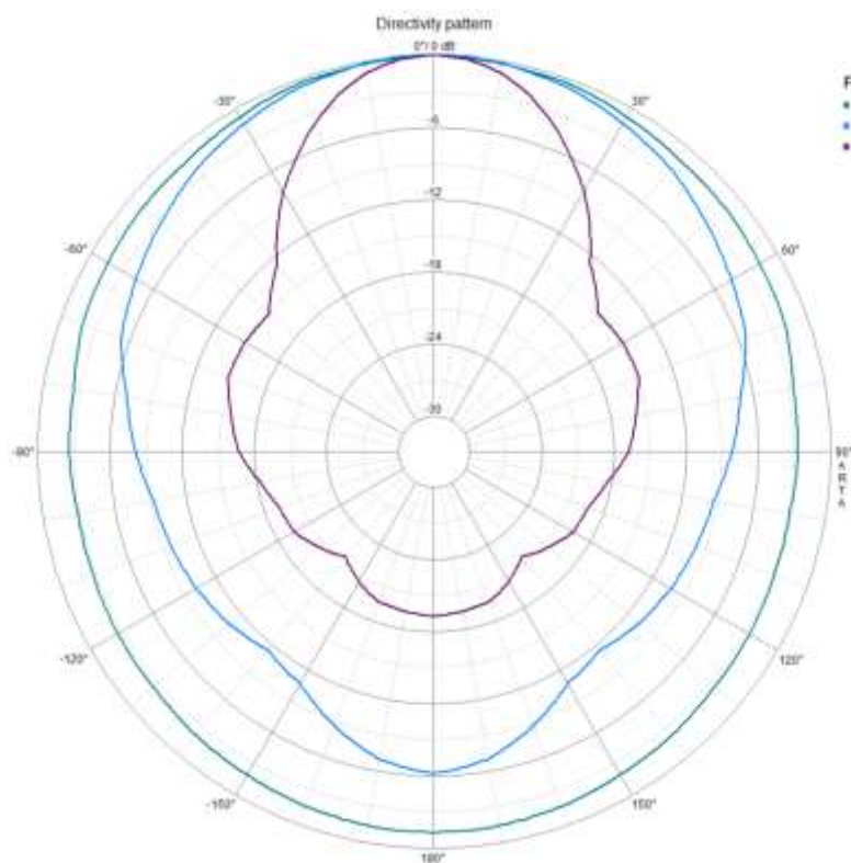
Abb. 6.2: Polardiagramm mit Abstrahlcharakteristik des Spötl-Lautsprechers
