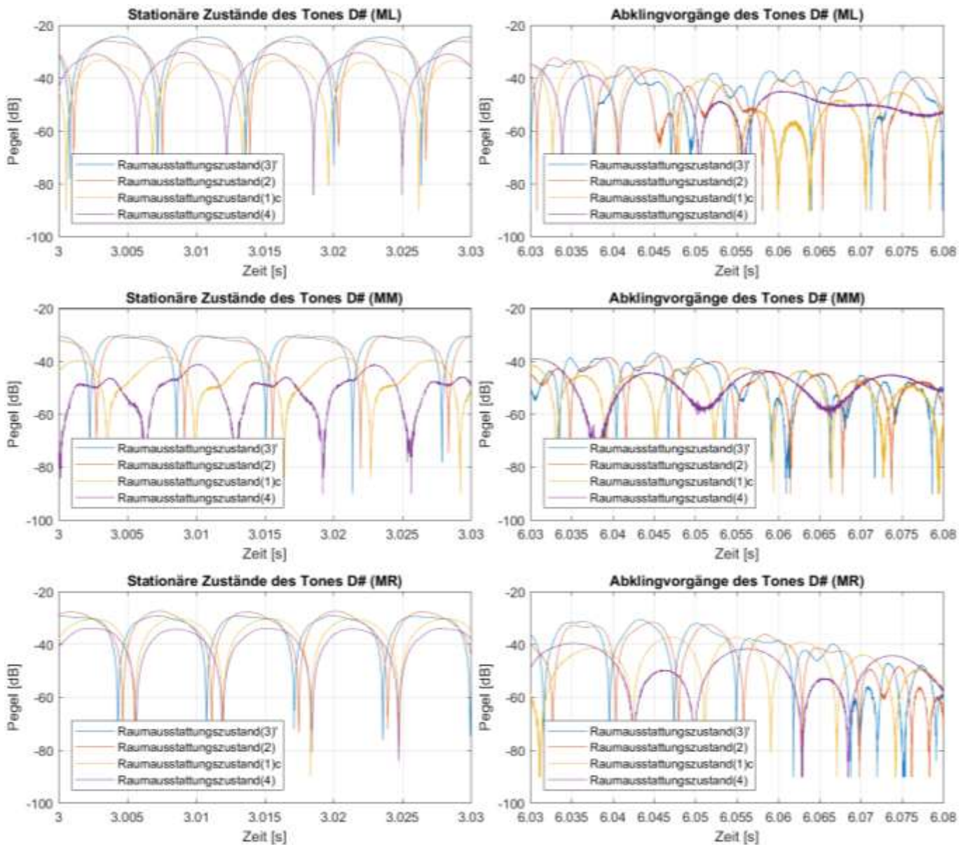
Abb. 6.24: Messsignalwellenformen der Marimbatonmessungen bei Anregung von Quellposition (Q1) mit der Grundfrequenz des Tones D# ( \cong 78 Hz) für alle vier Raumausstattungs Zustände (3)', (2), (1)c und (4) sowie die Mikrofonpositionen (ML), (MM) und (MR)
