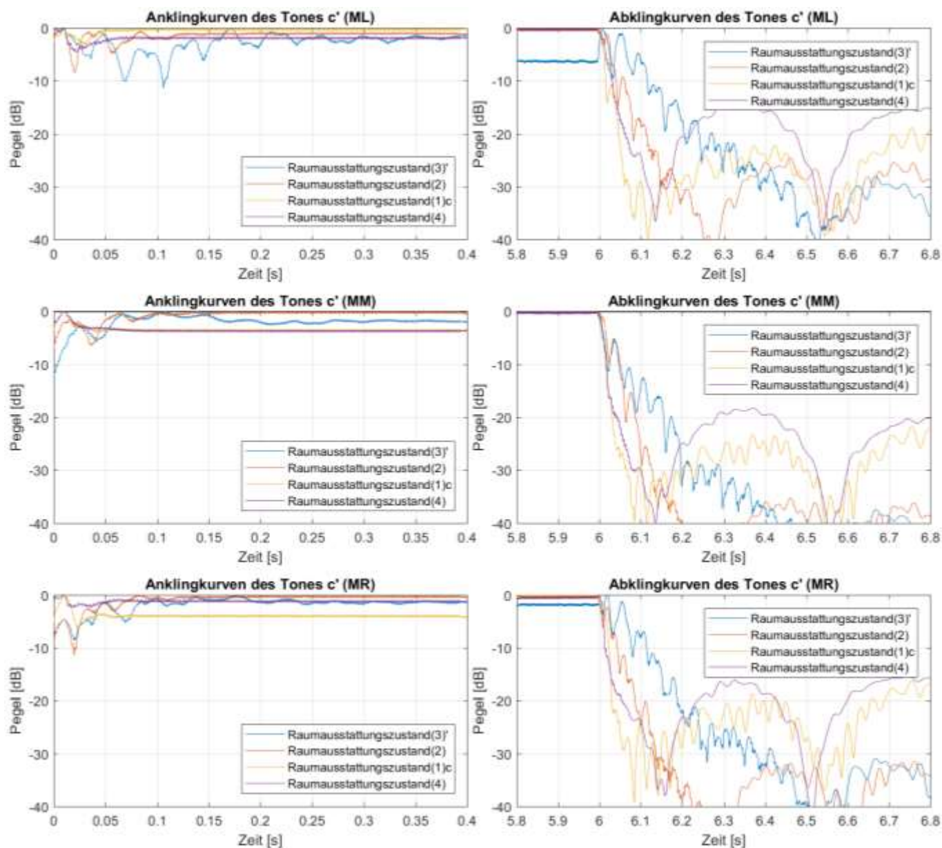
Abb. B1.25: An- und Abklingkurven der Marimbatonmessungen bei Anregung von Quellposition ( Q3 ) mit der Grundfrequenz des Tones c' ( \cong 263 Hz) für alle vier Raumausstattungs Zustände ( 3' ), ( 2 ), ( 1 )c und ( 4 ) sowie die Mikrofonpositionen ( ML ), ( MM ) und ( MR )
