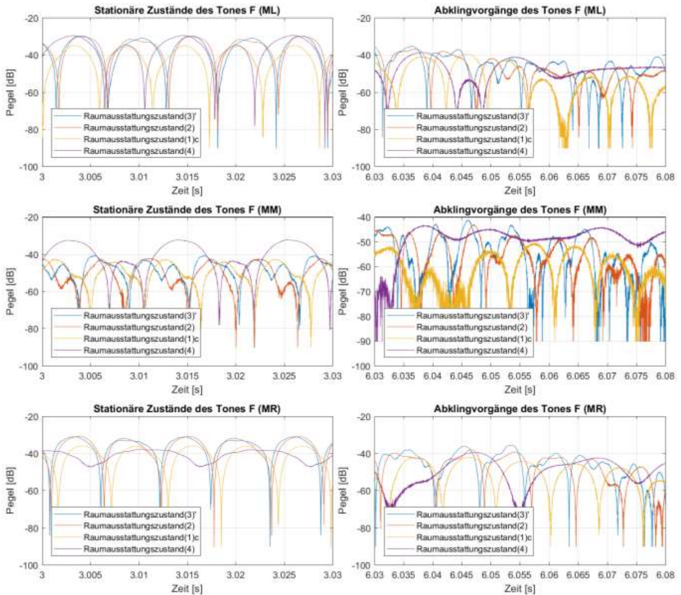
Abb. B2.6: Messsignalwellenformen der Marimbatonmessungen bei Anregung von Quellposition (Q1) mit der Grundfrequenz des Tones F ( \cong 88 Hz) für alle vier Raumausstattungs Zustände (3)', (2), (1)c und (4) sowie die Mikrofonpositionen (ML), (MM) und (MR)
