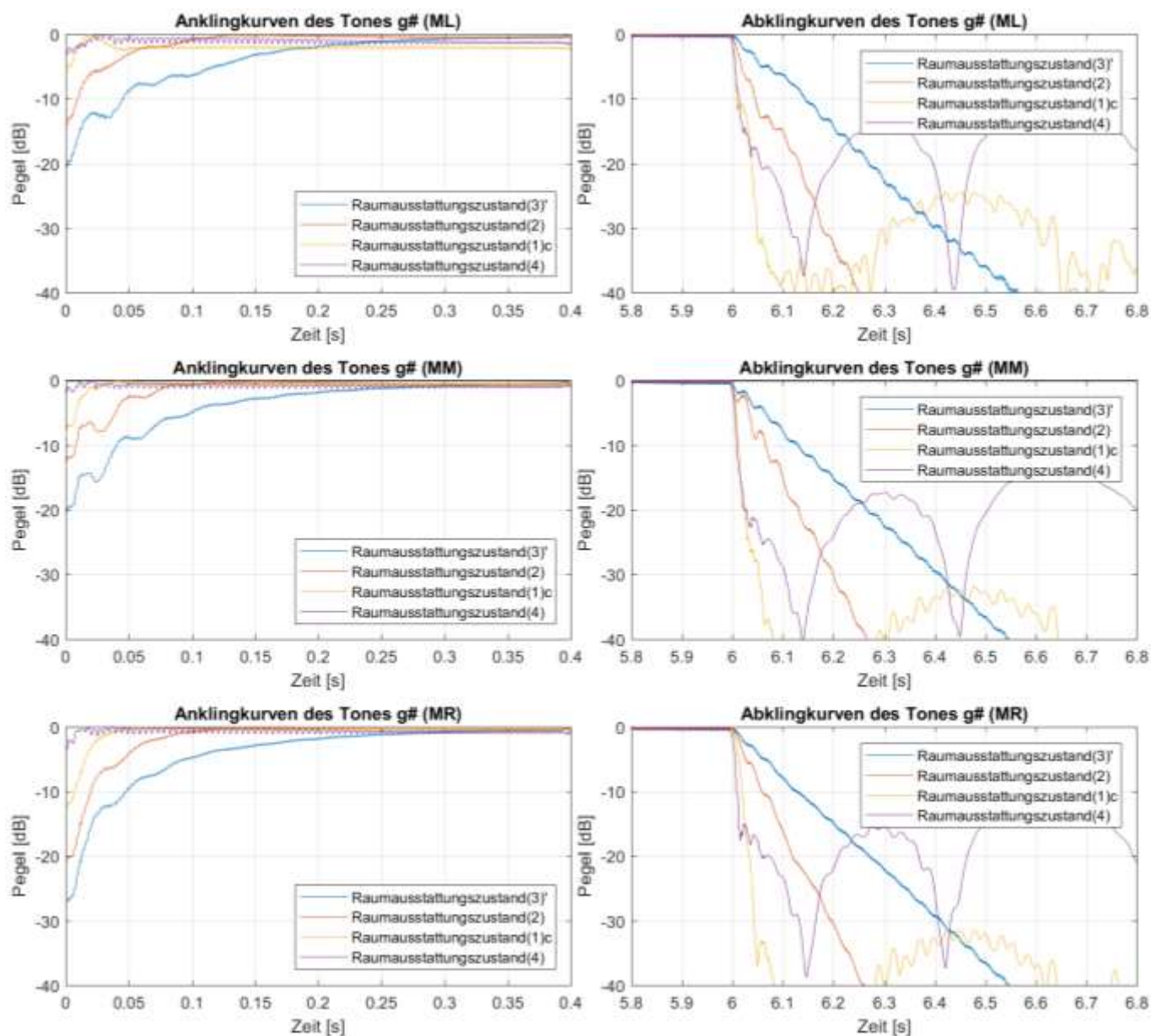
Abb. B1.21: An- und Abklingkurven der Marimbatonmessungen bei Anregung von Quellposition ( Q3 ) mit der Grundfrequenz des Tones g# ( \cong 209 Hz) für alle vier Raumausstattungs Zustände ( 3' ), ( 2 ), ( 1 )c und ( 4 ) sowie die Mikrofonpositionen ( ML ), ( MM ) und ( MR )
