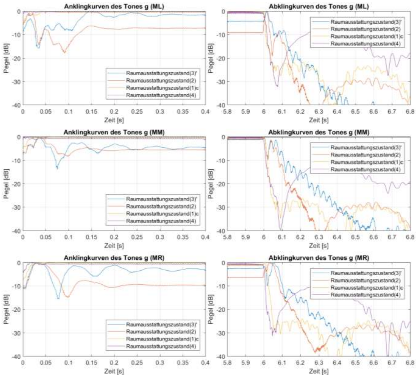
Abb. B1.20: An- und Abklingkurven der Marimbatonmessungen bei Anregung von Quellposition ( Q3 ) mit der Grundfrequenz des Tones g ( \cong 197 Hz) für alle vier Raumausstattungszustände ( 3' , (2) , (1)c und (4) sowie die Mikrofonpositionen ( ML ), ( MM ) und ( MR )
