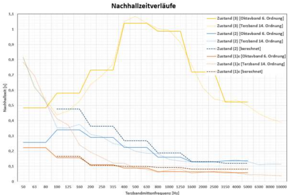
Abb. 5.17: Nachhallzeitverläufe für Raumausstattungs Zustände (1)c , (2) und (3) mit Oktavbandfilterung 6. Ordnung und Terzbandfilterung 14. Ordnung sowie Berechnung der Zustände (2) und (1)c aus (3) mit Oktavbandfilterung 6. Ordnung
