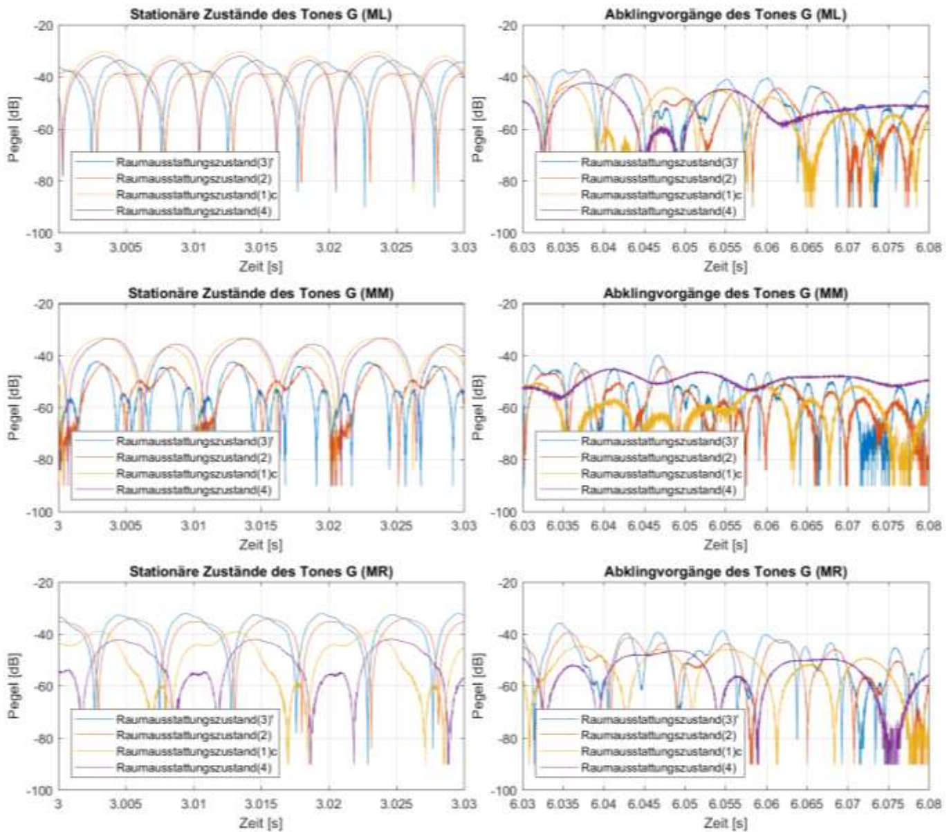
Abb. B2.8: Messsignalwellenformen der Marimbatonmessungen bei Anregung von Quellposition (Q1) mit der Grundfrequenz des Tones G ( \cong 99 Hz) für alle vier Raumausstattungszustände (3), (2), (1)c und (4) sowie die Mikrofonpositionen (ML), (MM) und (MR)
