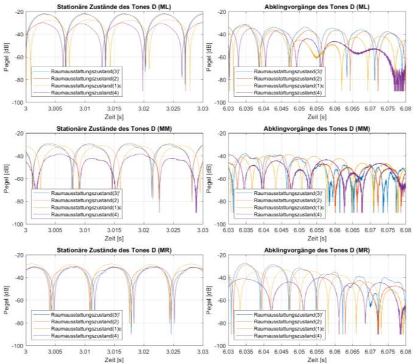
Abb. B2.3: Messsignalwellenformen der Marimbatonmessungen bei Anregung von Quellposition ( Q1 ) mit der Grundfrequenz des Tones D ( \hat{=} 74 Hz) für alle vier Raumausstattungsstände ( 3 ) j , ( 2 ), ( 1 ) c und ( 4 ) sowie die Mikrofonpositionen ( ML ), ( MM ) und ( MR )
