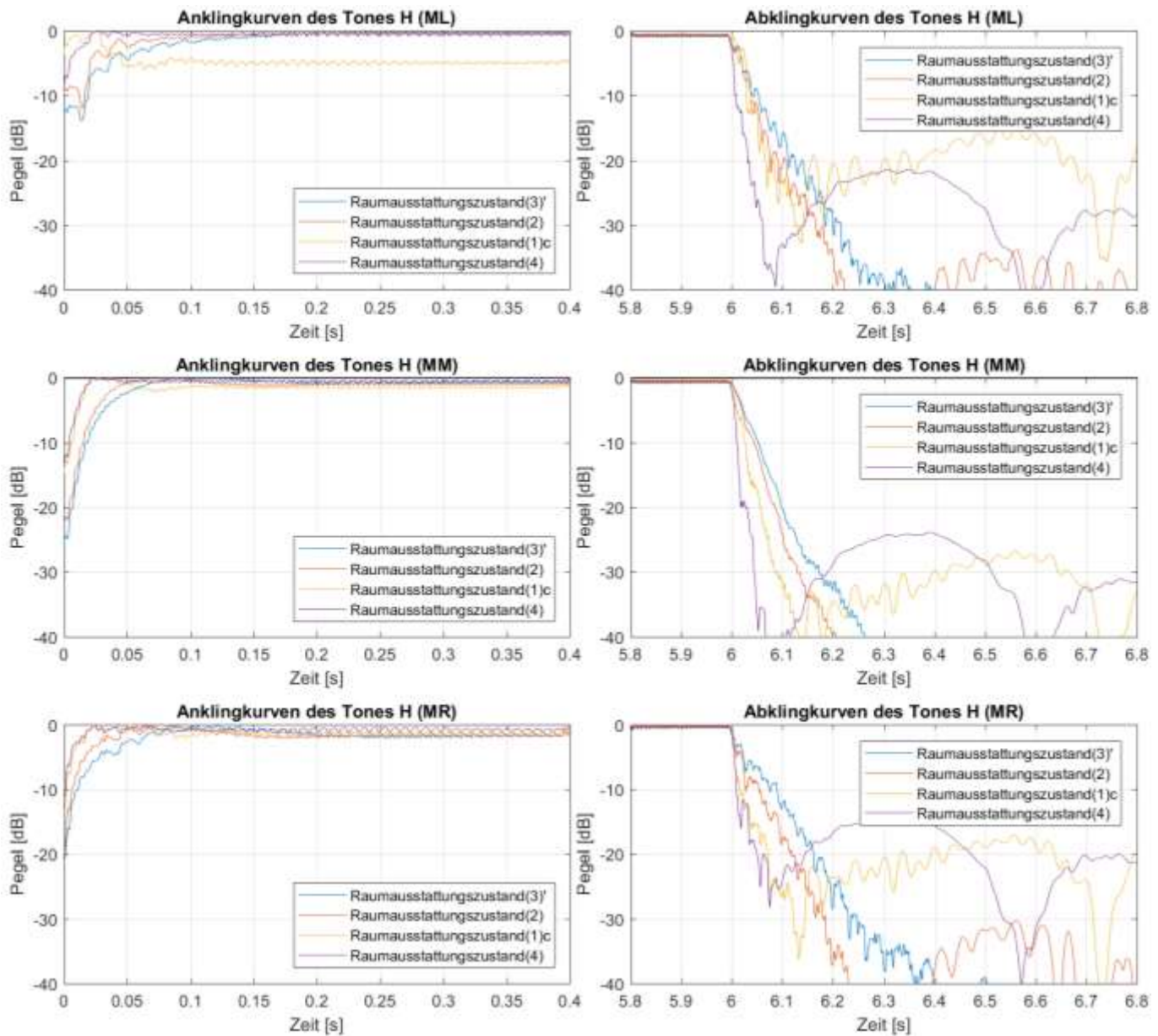
Abb. B1.12: An- und Abklingkurven der Marimbatonmessungen bei Anregung von Quellposition (Q2) mit der Grundfrequenz des Tones H ( \cong 124 Hz) für alle vier Raumausstattungszustände (3)', (2), (1)c und (4) sowie die Mikrofonpositionen (ML), (MM) und (MR)
