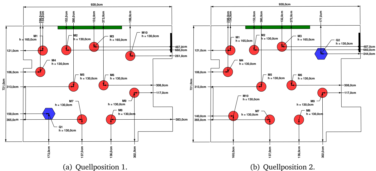
Abbildung A.0.3: Skizze der Mikrofon- bzw. Quellpositionen.
