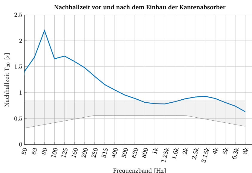
Abbildung 2.1: Nachhallzeitverlauf im FSI2. Grauer Bereich kennzeichnet den Bereich idealer Nachhallzeit nach ÖNORM B 8115-3.
