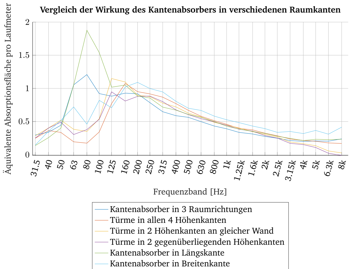
Abbildung 3.2: Vergleich der Wirkung des Kantenabsorbers bei Aufstellungen in verschiedenen Kanten im Hallraum (Länge 8,35 m, Breite 5,99 m, Höhe 4,90 m).
