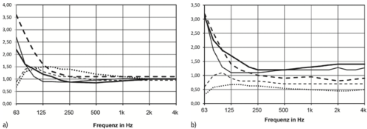
Abbildung 3.1: a) Absorptionsgrad \alpha bezogen auf die gesamte Oberfläche bzw. b) Absorptionsfläche A in \text{m}^2 bezogen auf die Kantenlänge in \text{m}/\text{m}^2 von Kantenabsorbern mit verschiedenen Querschnitten; dicke Linie: 400\text{ mm} \times 1000\text{ mm} ; dünne Linie: 200\text{ mm} \times 1000\text{ mm} ; dick strichliert: 400\text{ mm} \times 500\text{ mm} ; dünn strichliert: 200\text{ mm} \times 500\text{ mm} ; punktiert: 200\text{ mm} \times 250\text{ mm}
