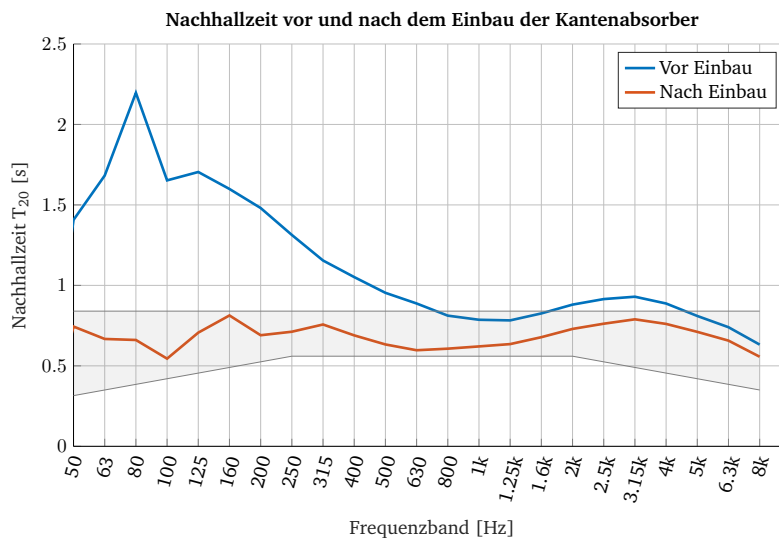
Abbildung 2.5: Nachhallzeit vor und nach dem Einbau im FS12. Grauer Bereich kennzeichnet den Bereich idealer Nachhallzeit nach ÖNORM B 8115-3.
