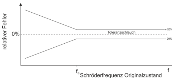
Abbildung 7.3: Schematische, qualitative Darstellung eines Toleranzschlauches für eine zu erfüllende, normgerechte Nachhallzeit.
