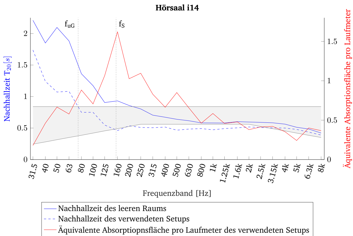
Abbildung 3.14: Nachhallzeit ( T_{20} ) und äquivalente Absorptionsfläche pro Laufmeter im Hörsaal i14.
