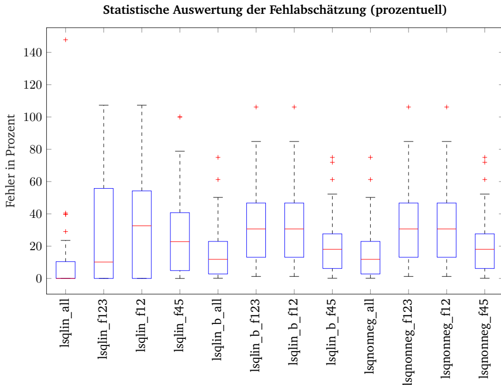
Abbildung 5.2: Statistische Auswertung der Fehlabschätzung in Prozent für die verschiedenen verwendeten Algorithmen.
