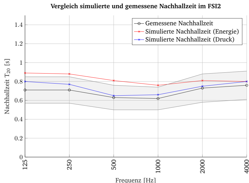
Abbildung 7.9: Vergleich zwischen simulierter und gemessener Nachhallzeit im FS12. Grauer Bereich stellt den Bereich von \pm 20 Prozent des gemessenen Wertes dar.
