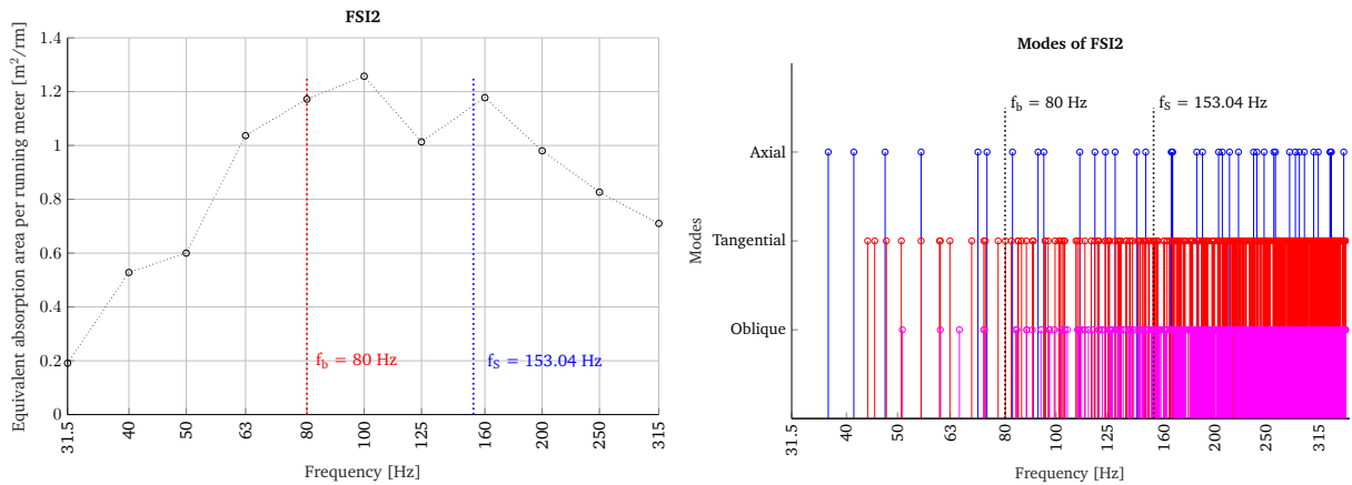
(a) Berechneter Verlauf der Äquivalente Absorptionsfläche im FS12.
