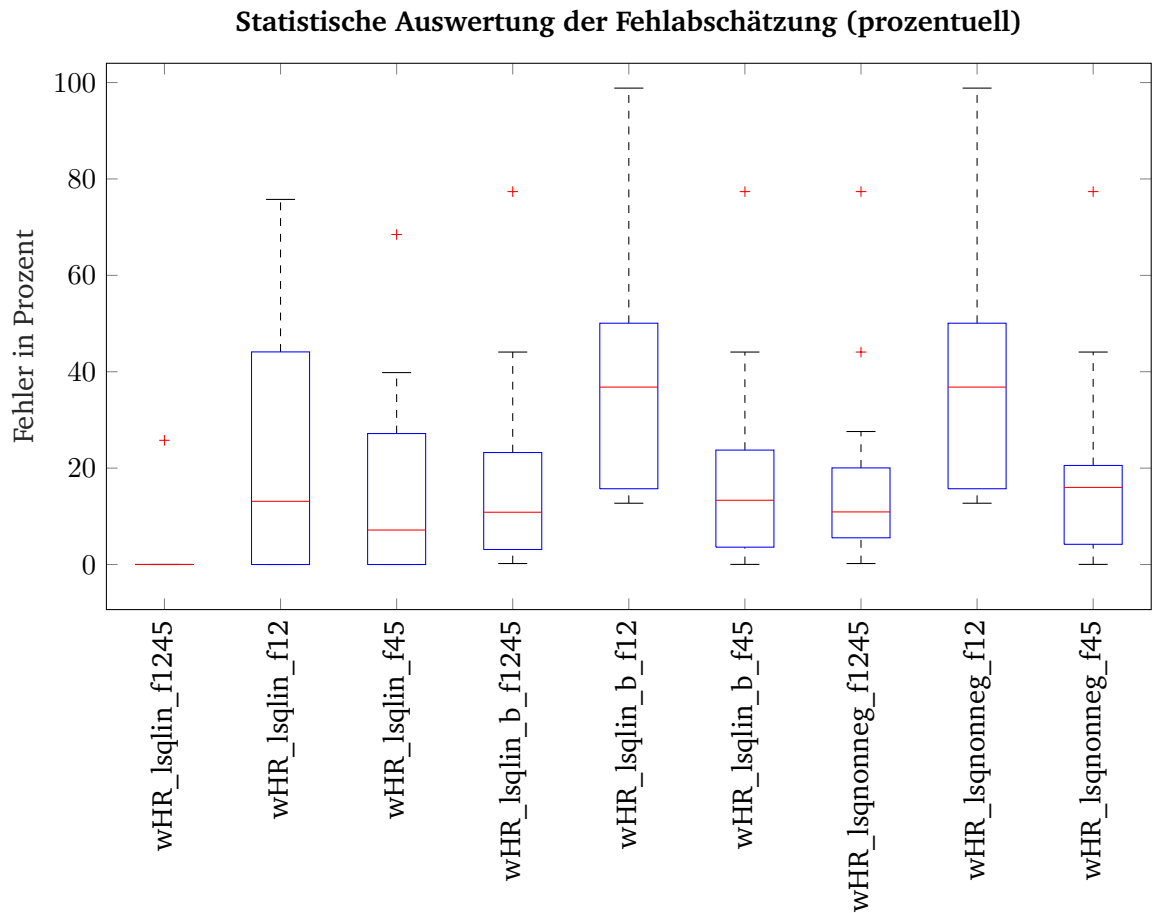
Abbildung 5.4: Statistische Auswertung der Fehlabschätzung in Prozent für die verwendeten Algorithmen ohne Berücksichtigung des Hallraums.
