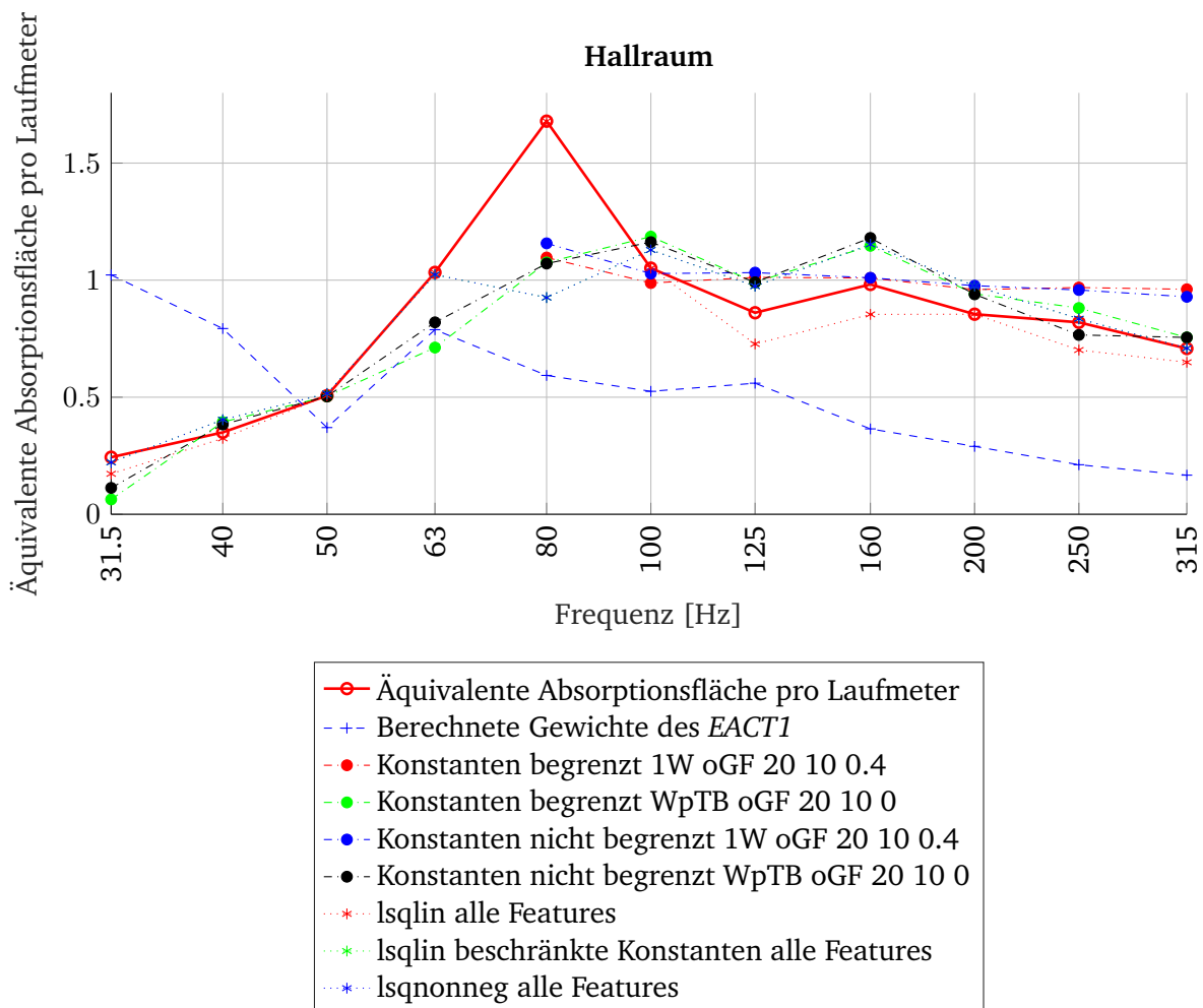
Abbildung 6.1: Ergebnisse der durchgeführten Optimierungen im Hallraum.
