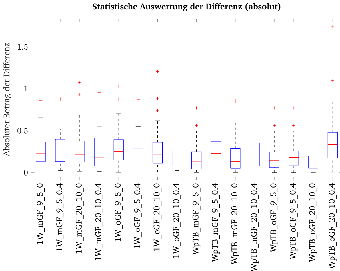
Abbildung 4.5: Statistische Auswertung der Differenz der Optimierungen des EACT1 mit Beschränkung der Konstanten.
