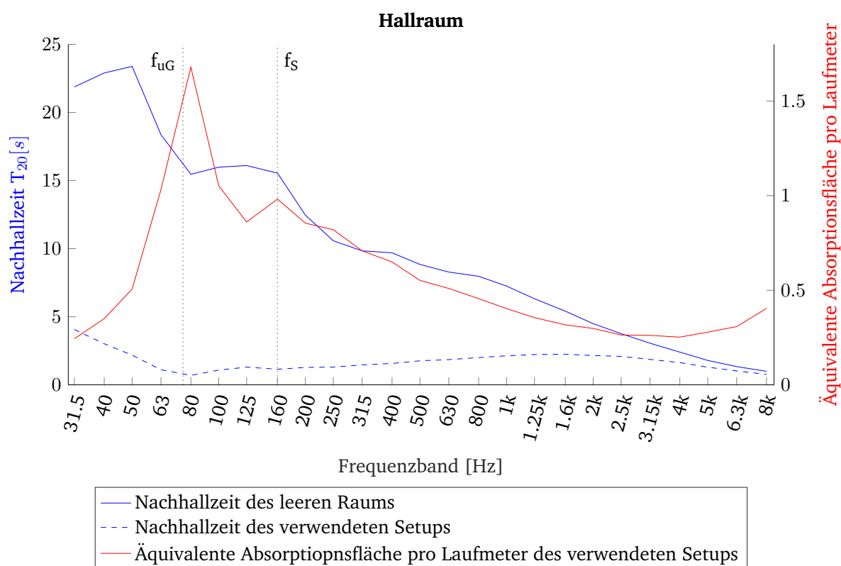
Abbildung 3.5: Nachhallzeit ( T_{20} ) und äquivalente Absorptionsfläche pro Laufmeter im Hallraum.
