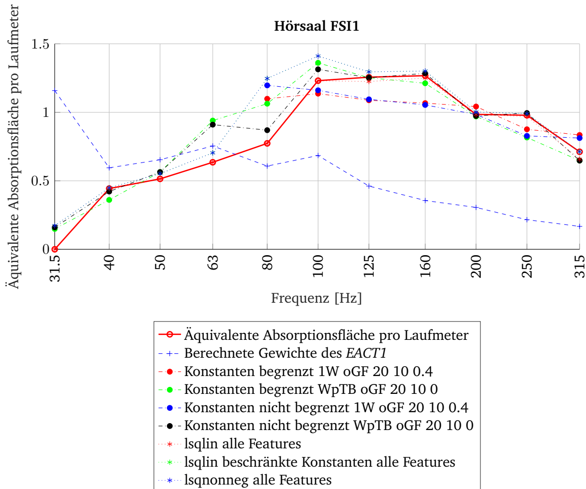
Abbildung 6.3: Ergebnisse der durchgeführten Optimierungen im Hörsaal FS11.
