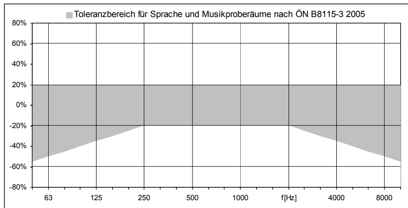
Abbildung 1.2: Toleranzbereich der Nachhallzeit für Sprache und Musikproberäume nach ÖNORM B 8115-3.
