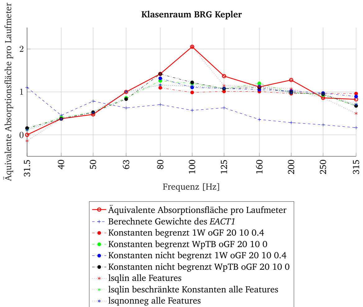
Abbildung 6.2: Ergebnisse der durchgeführten Optimierungen im Klassenraum des BRG Kepler.
