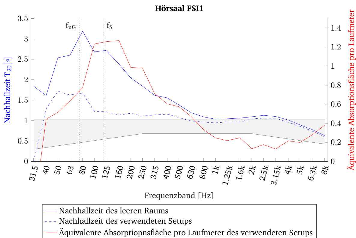
Abbildung 3.9: Nachhallzeit ( T_{20} ) und äquivalente Absorptionsfläche pro Laufmeter im Hörsaal FSI1.
