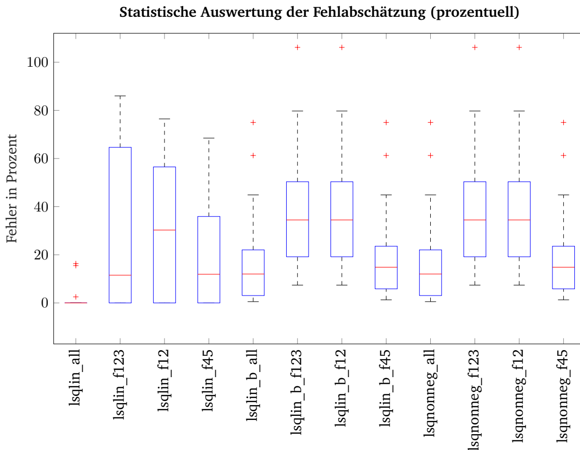
Abbildung 5.3: Statistische Auswertung der Fehlabschätzung in Prozent für die verschiedenen verwendeten Algorithmen im Terzbandbereich von 63 bis 125 Hz.
