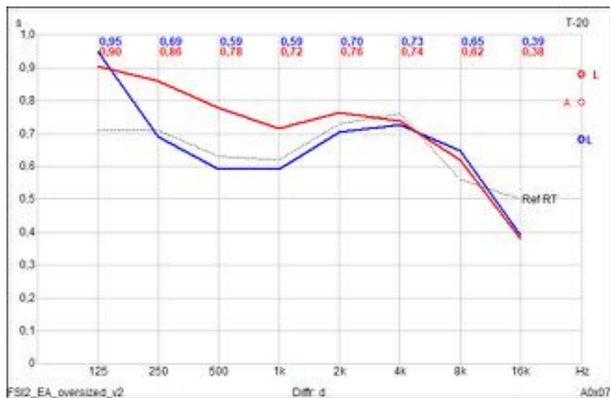
Abbildung 7.6: Vergleich rote und blaue Kurve anhand Messposition 7 bei Simulation mit dem vergrößerten Absorber.
