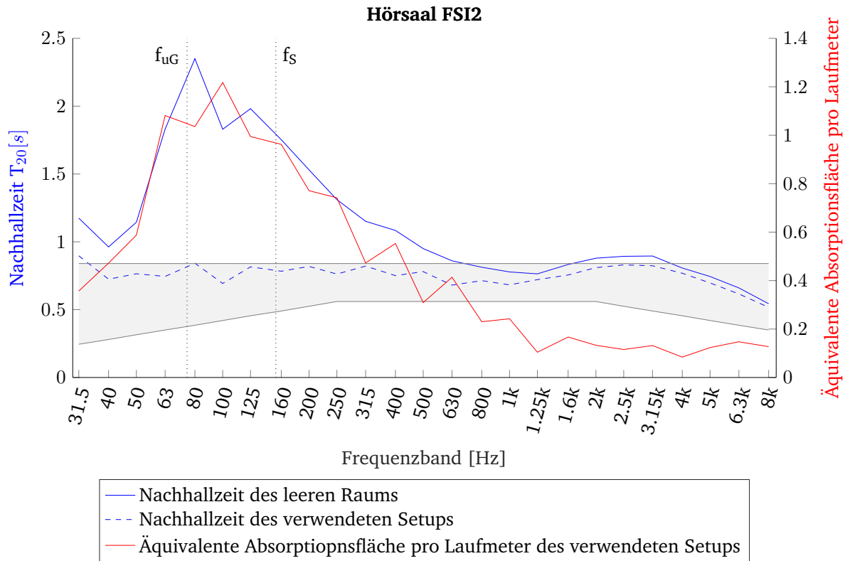
Abbildung 3.11: Nachhallzeit ( T_{20} ) und äquivalente Absorptionsfläche pro Laufmeter im Hörsaal FSI2.
