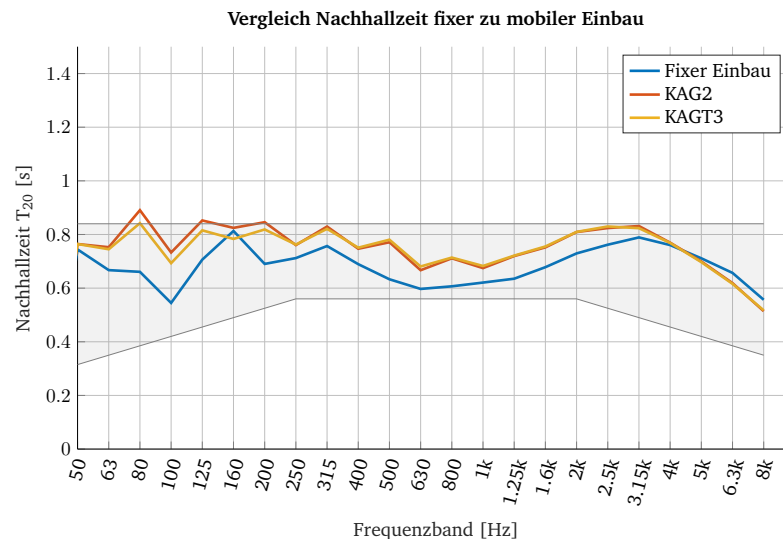
Abbildung 2.8: Vergleich der Nachhallzeit des fixen Einbaus im Vergleich zu den beiden Setups der mobilen Messung. Grauer Bereich kennzeichnet den Bereich idealer Nachhallzeit nach ÖNORM B 8115-3.
