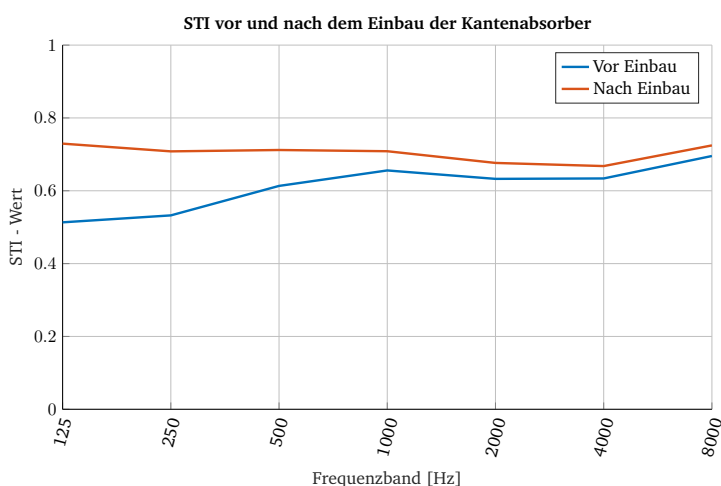
Abbildung 2.6: STI vor und nach dem Einbau im FSI2
