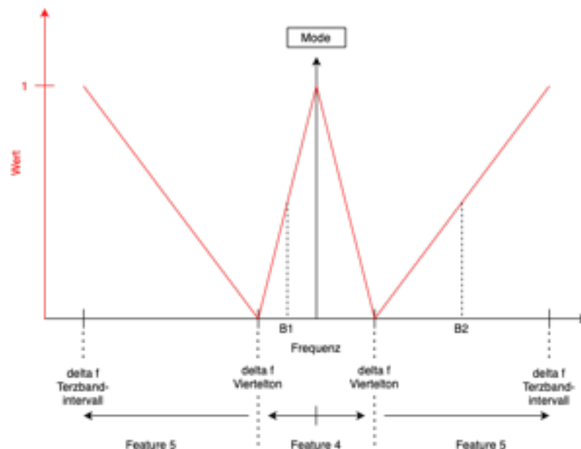
Abbildung 5.1: Grafik zu Feature 4 und 5. Die strichliert angedachten Moden B1 und B2 würden beide den Wert 0,5 bewirken. B1 im Feature 4, B2 im Feature 5.
