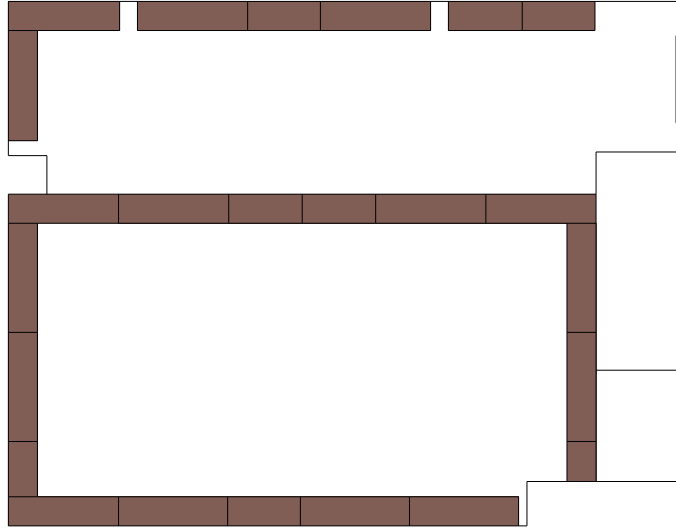
Abbildung 2.2: Skizze der Kantenabsorber, angebracht an der Decke im Hörsaal FSI2.
