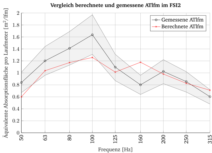
Abbildung 7.8: Vergleich zwischen berechneter und gemessener äquivalenter Absorptionsfläche im FSI2. Grauer Bereich stellt den Bereich von \pm 20 Prozent des gemessenen Wertes dar.
