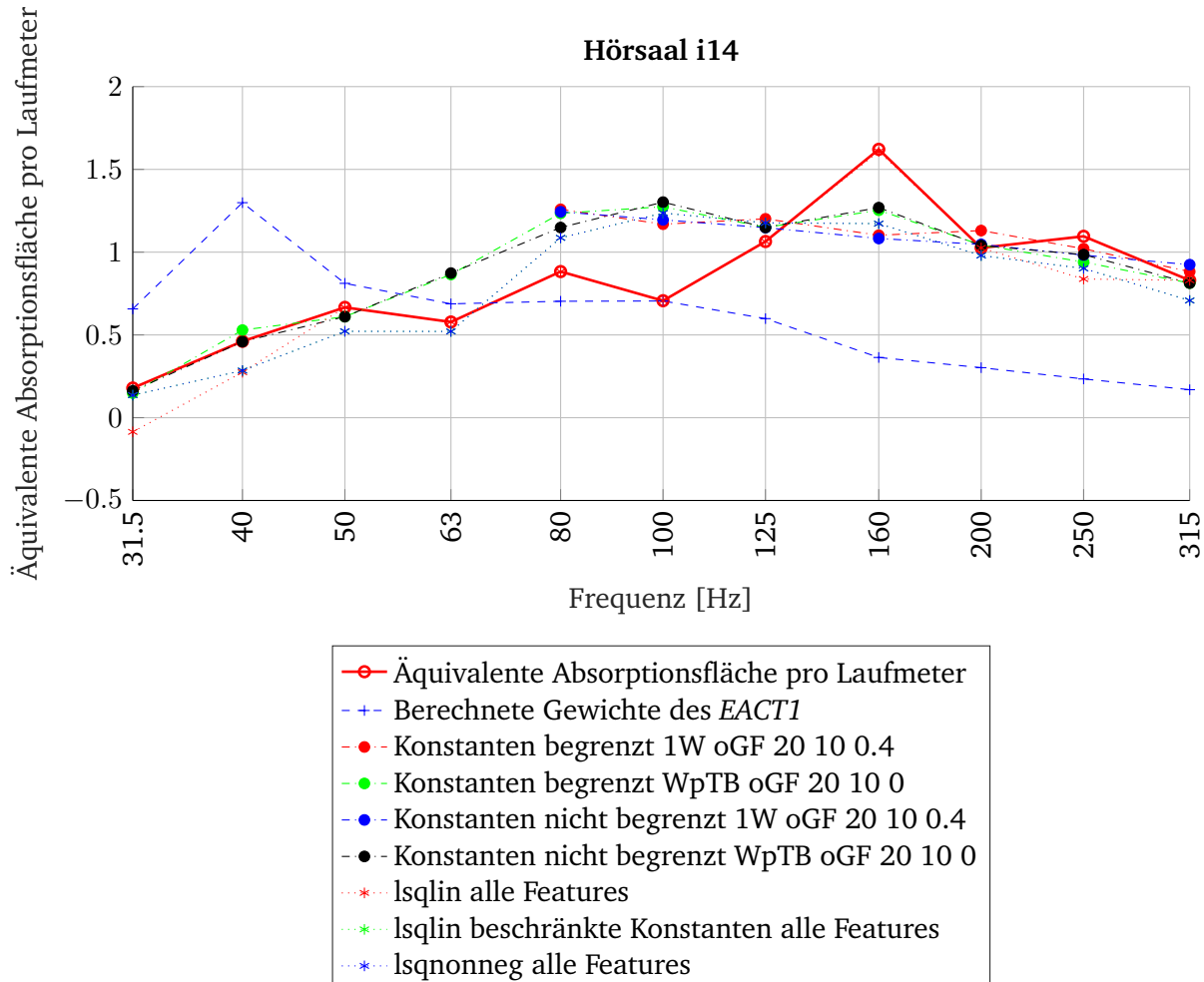
Abbildung 6.5: Ergebnisse der durchgeführten Optimierungen im Hörsaal i14.
