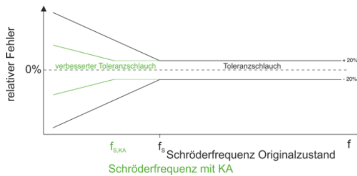
Abbildung 7.4: Verbesserter Toleranzschlauch durch akustische Maßnahme.
