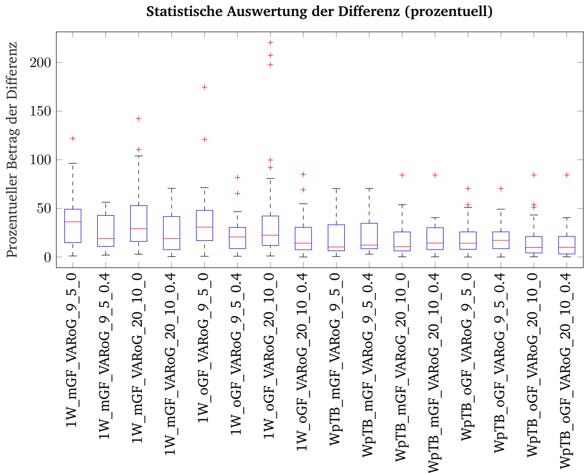
Abbildung 4.7: Statistische Auswertung der Differenz der Optimierungen des EACT1 ohne Beschränkung der Konstanten normiert in Prozent.
