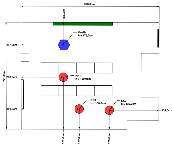
(a) Aufstellungsplan.
