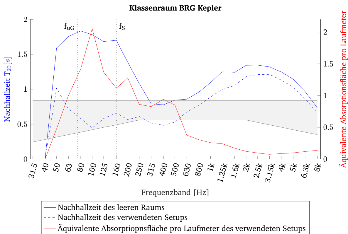
Abbildung 3.7: Nachhallzeit ( T_{20} ) und äquivalente Absorptionsfläche pro Laufmeter im Klassenraum des BRG Kepler.
