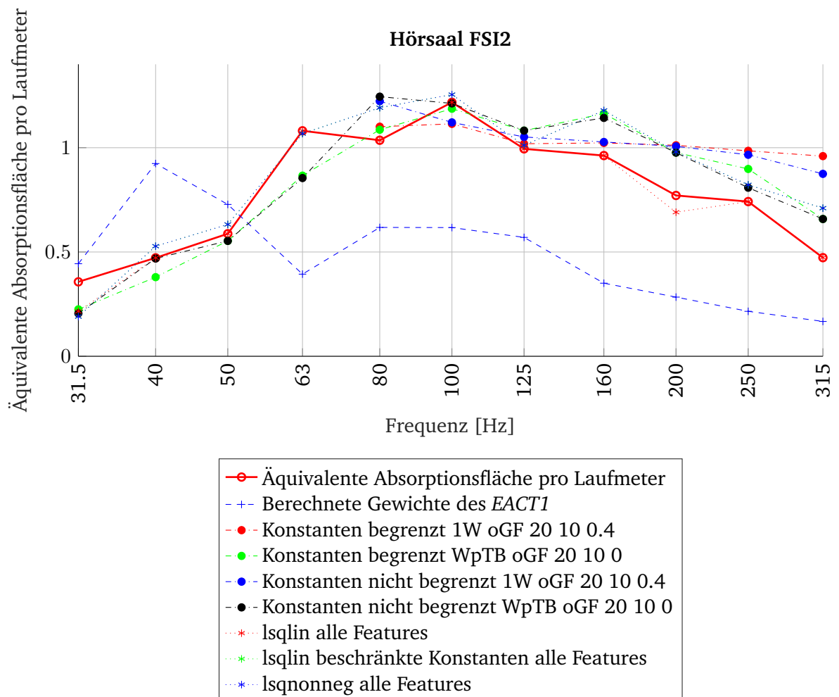
Abbildung 6.4: Ergebnisse der durchgeführten Optimierungen im Hörsaal FSI2.
