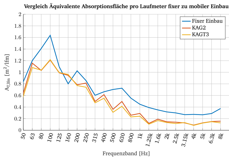
Abbildung 2.9: Vergleich der äquivalenten Absorptionsfläche pro Laufmeter Kantenabsorber des fixen Einbaus im Vergleich zu den beiden Setups der mobilen Messung.
