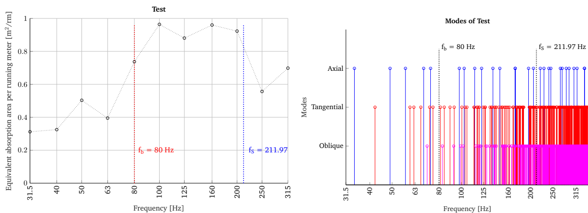
(a) Von EACT2 berechnete Äquivalente Absorptionsfläche in Abhängigkeit von der Raummodenverteilung.
