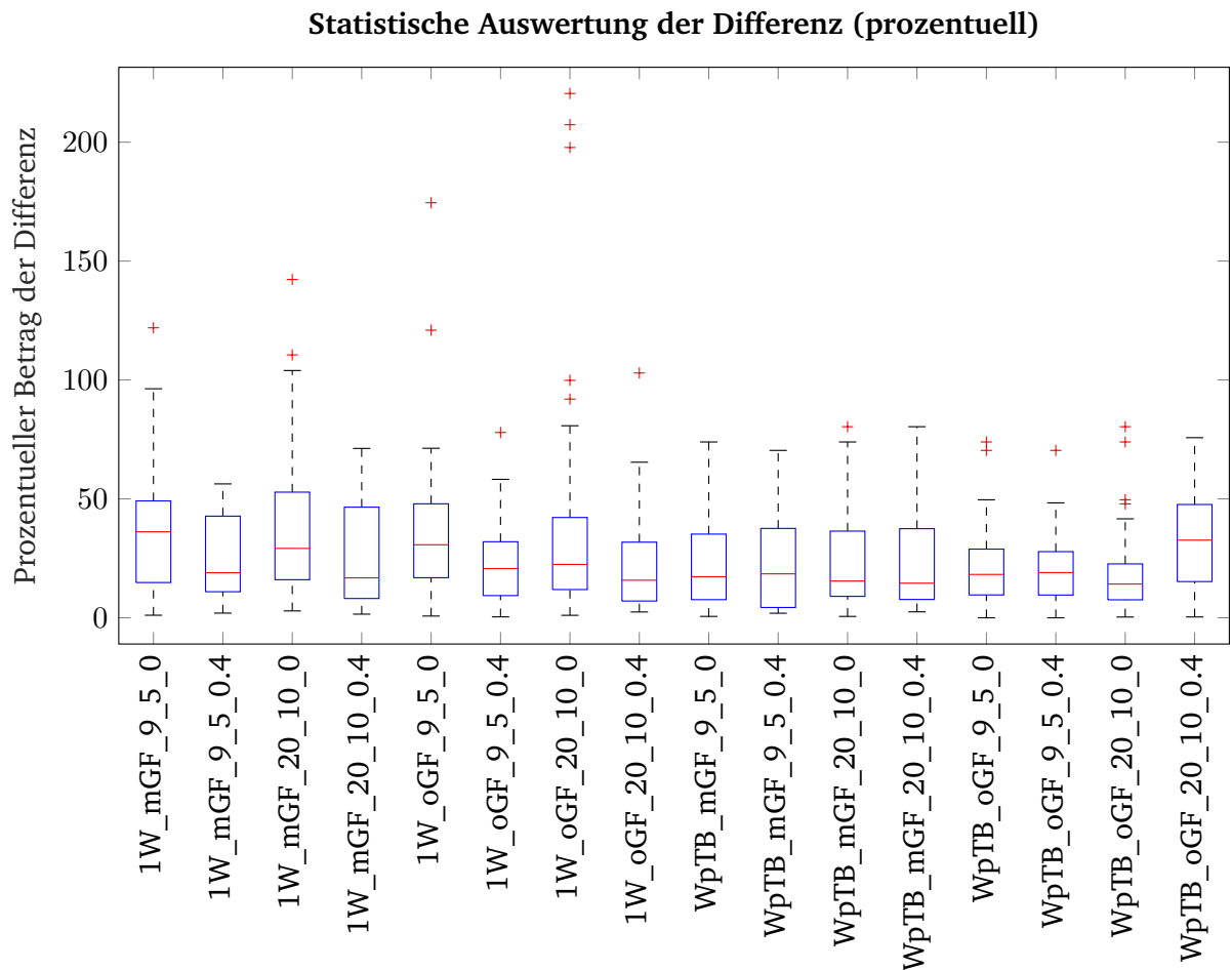
Abbildung 4.6: Statistische Auswertung der Differenz der Optimierungen des EACT1 mit Beschränkung der Konstanten normiert in Prozent.
